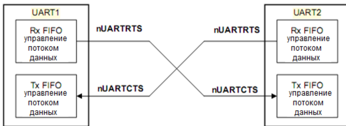
Рисунок 98 – Взаимодействие двух устройств последовательной связи с аппаратным управлением потоком данных
