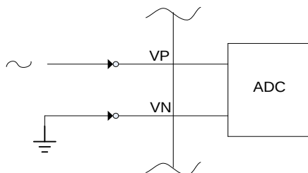
Рисунок 32 – Недифференциальное включение
