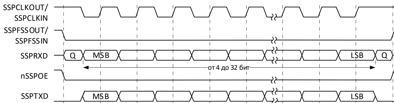
Рисунок 85 – Формат синхронного обмена протокола SPI, SPO=1, SPH=1
