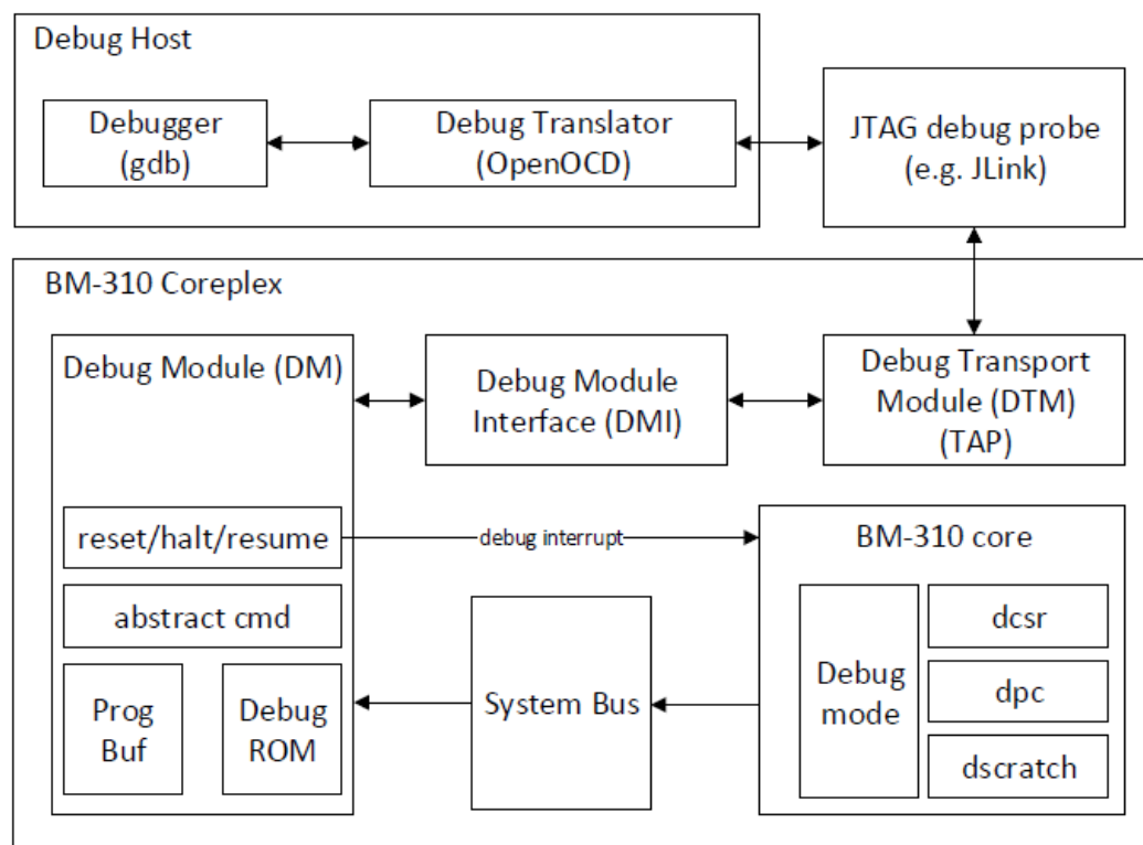
Рисунок 112 – Архитектура системы отладки
