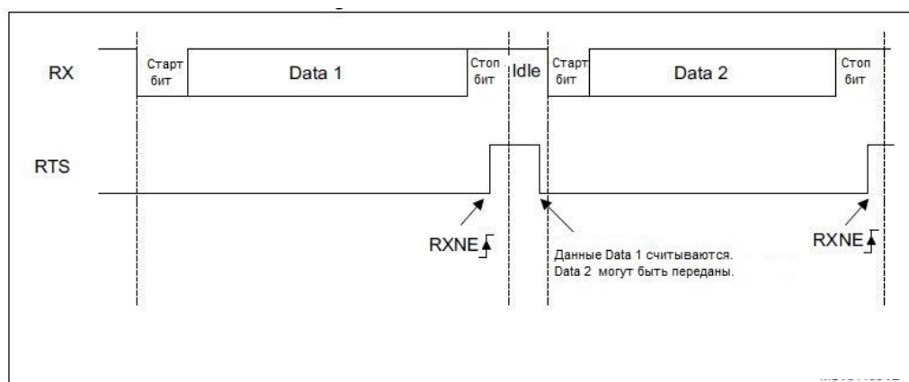
Рисунок 135 – Управление потоком RTS
