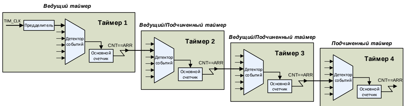
Рисунок 55 – Пример каскадного соединения таймеров
