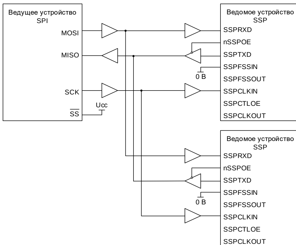
Рисунок 91 – Ведущее устройство, протокол SPI, подключено к двум ведомым модулям SSP
