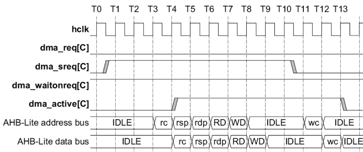
Рисунок 105 – Работа DMA при использовании dma_waitonreq совместно с dma_sreq
