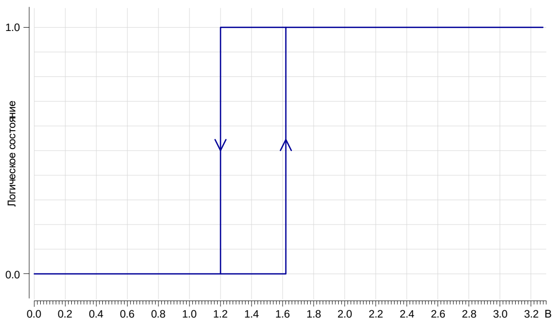
Рисунок 143 – Типовая зависимость логического состояния от напряжения на цифровом входе порта ввода-вывода при U_{CC} = 3,3 В в НУ
