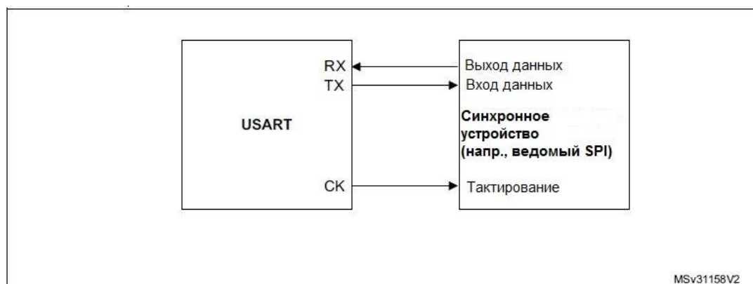
Рисунок 128 – Пример синхронной передачи USART
