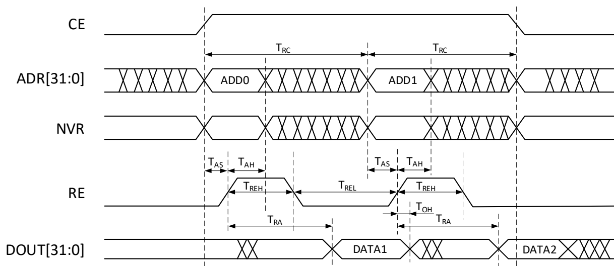
Рисунок 25 – Временная диаграмма чтения памяти
