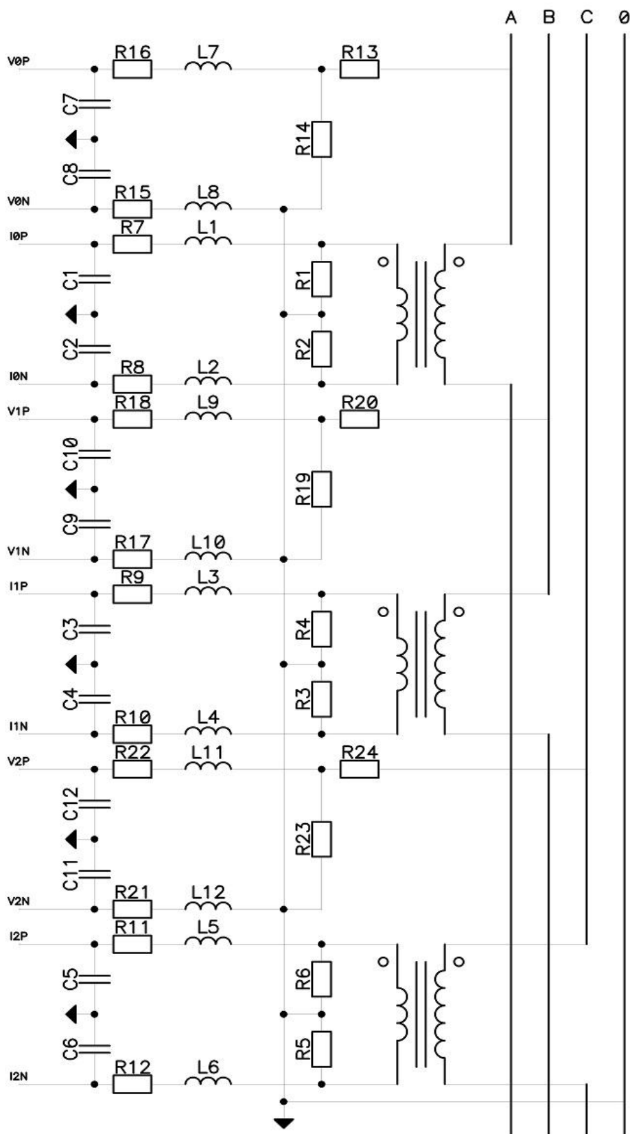
Рисунок 37 – Типовая схема включения для учета электроэнергии по трем фазам
