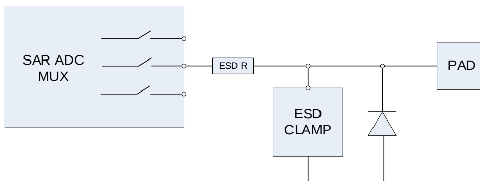
Рисунок 75 – Структурная схема выводов SAR_AINx
