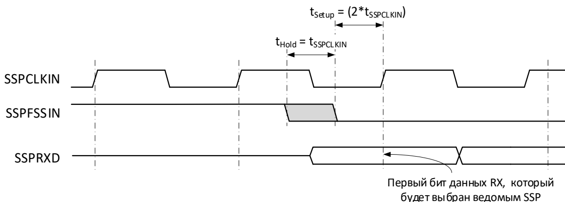
Рисунок 88 – Формат Microwire, требования к времени установки и удержания сигнала SSPFSSIN
