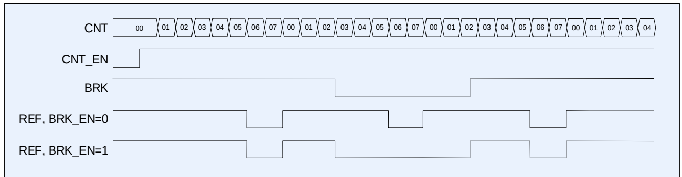
Рисунок 67 – Диаграмма сброса сигнала REF по выводу BRK
