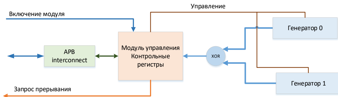
Рисунок 118 – Структурная схема блока генератора случайных чисел
