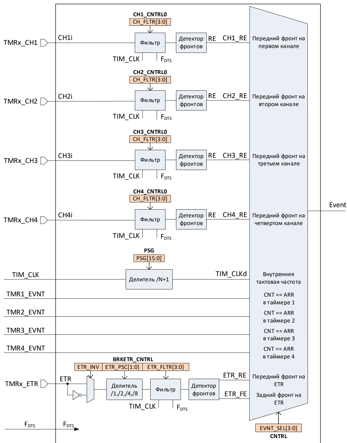
Рисунок 52 – Структурная схема формирования события для счета
