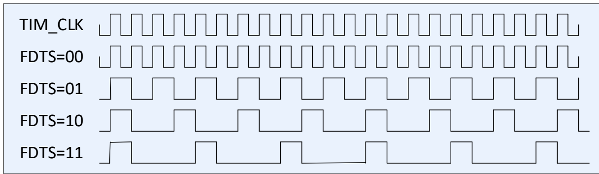
Рисунок 51 – Диаграмма тактовой частоты F_{DTS} в зависимости от значения FDTs[1:0] в регистре CNTRL
