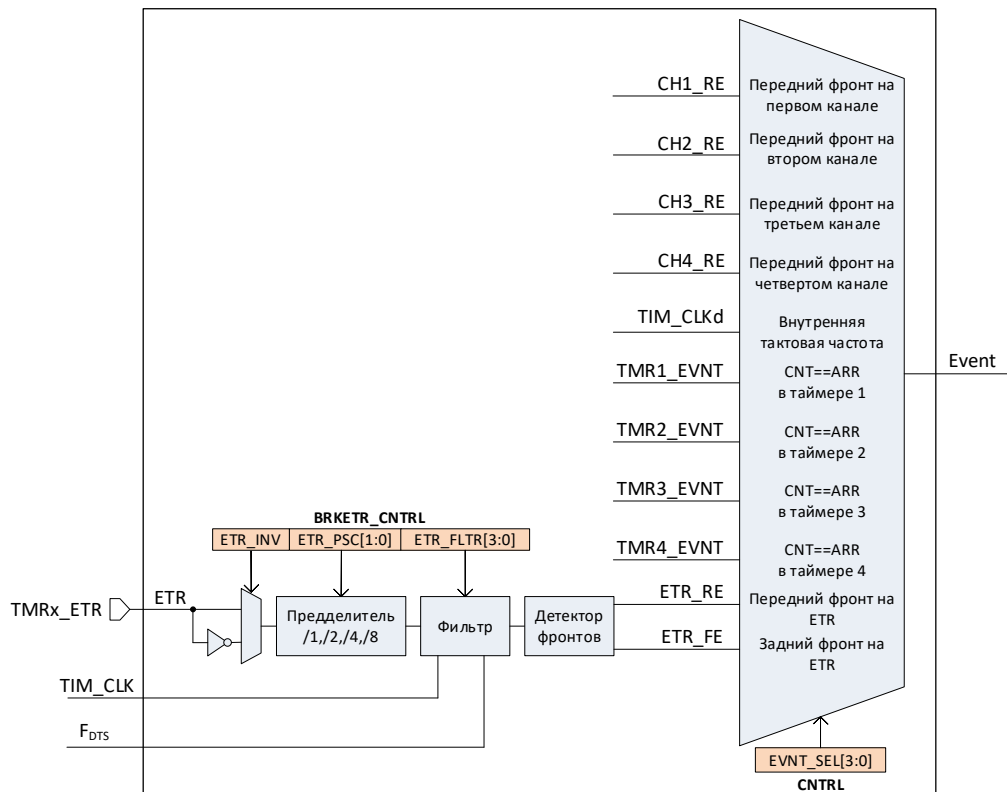
Рисунок 59 – Схема тактирования сигналом со входа ETR
