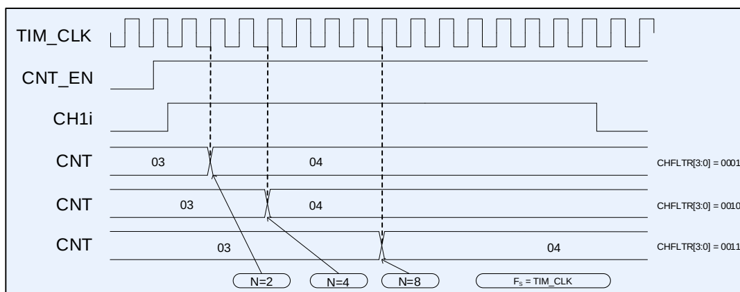
Рисунок 58 – Диаграмма внешнего тактирования с разными вариантами фильтра
