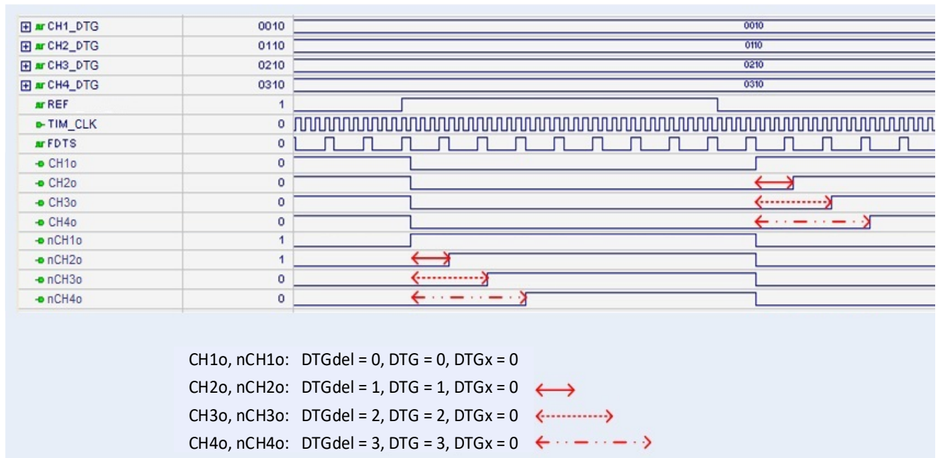
Рисунок 68 – Диаграмма работы блока DTG
