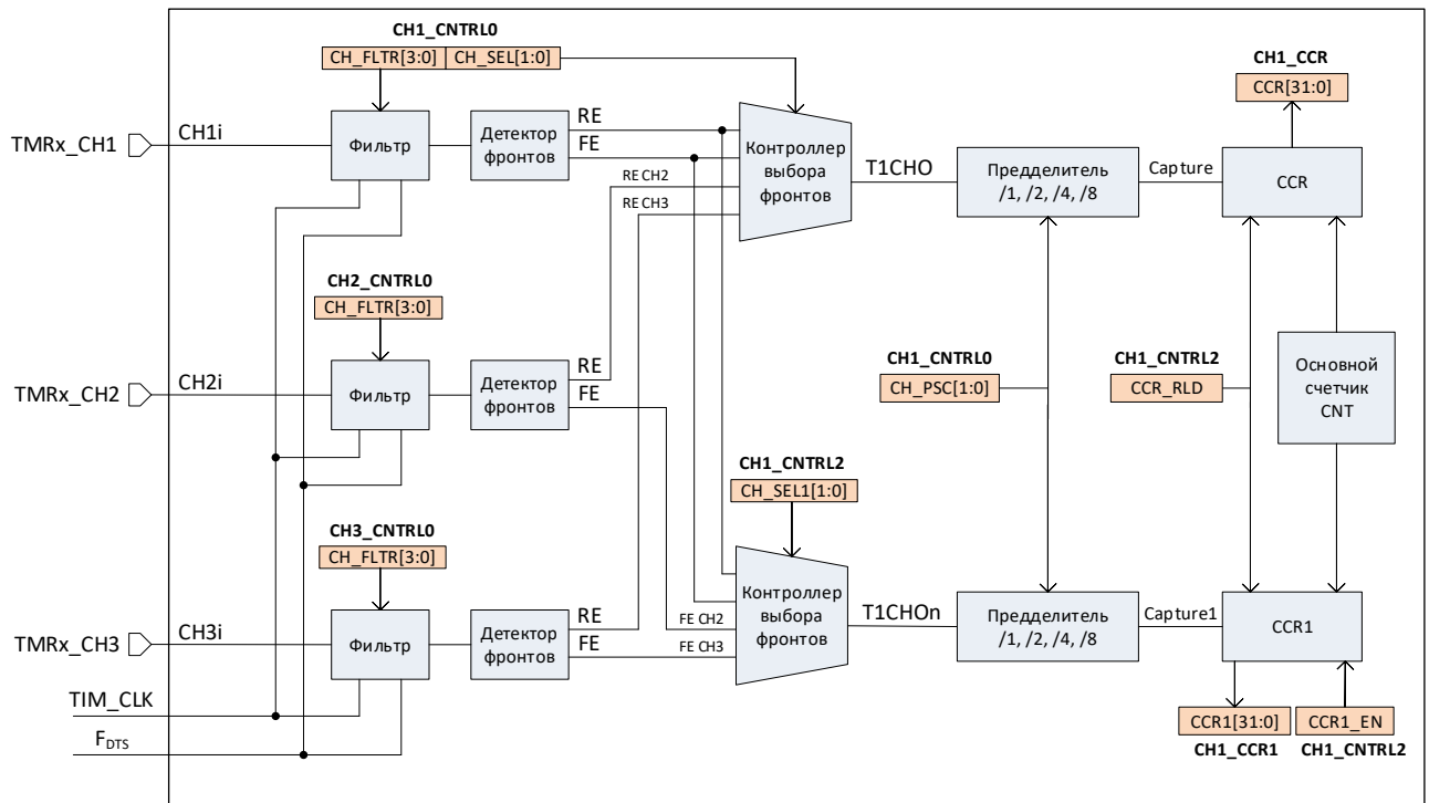
Рисунок 61 – Структурная схема блока захвата на примере канала 1
