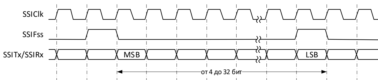
Рисунок 79 – Формат синхронного обмена протокола SSI (непрерывный обмен)
