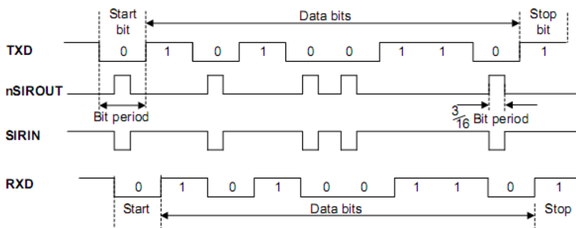
Рисунок 97 – Модуляция данных IrDA
