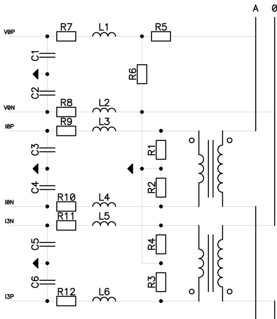
Рисунок 38 – Типовая схема включения для учета электроэнергии по одной фазе
