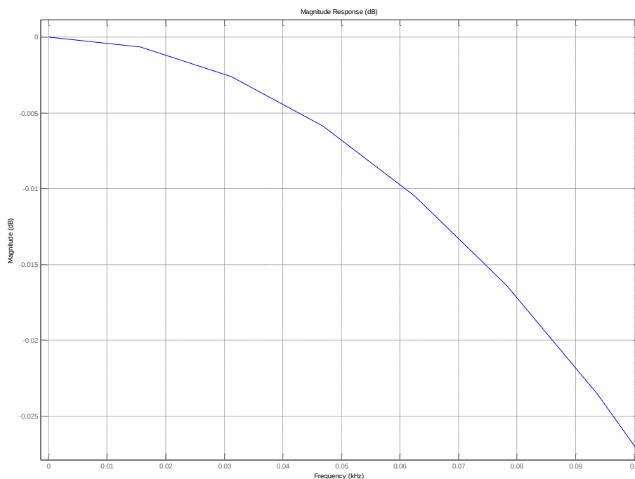
Рисунок 35 – Характеристика децимирующего фильтра в полосе 100 Гц
