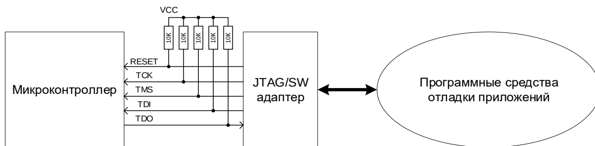
Рисунок 114 – Схема работы в режиме отладки
