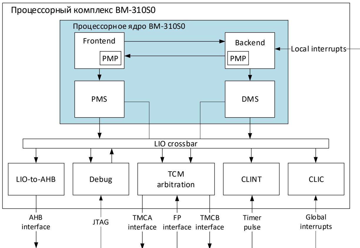
Рисунок 26 – Структурная схема процессора
