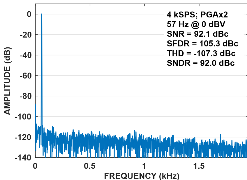
Рисунок 138 – Типовой спектр в НУ для \Delta\Sigma АЦП микросхем MDR1206FI (CHIP_ID = 217) в канале F2IDAT для дифференциального входного сигнала +/- 1 В (0.707 RMS). Усиление = 6 дБ (F2IGAIN = 00)
