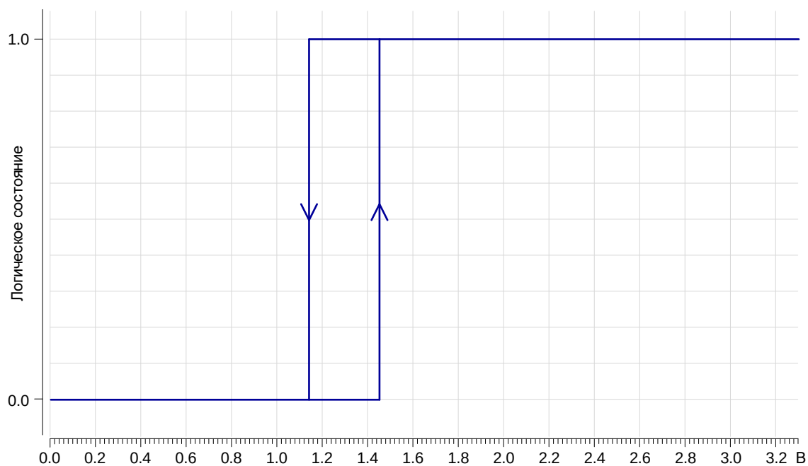
Рисунок 144 – Типовая зависимость логического состояния от напряжения на входе WAKEUP1-WAKEUP3 при U_{CCB} = 3,3 В в НУ
