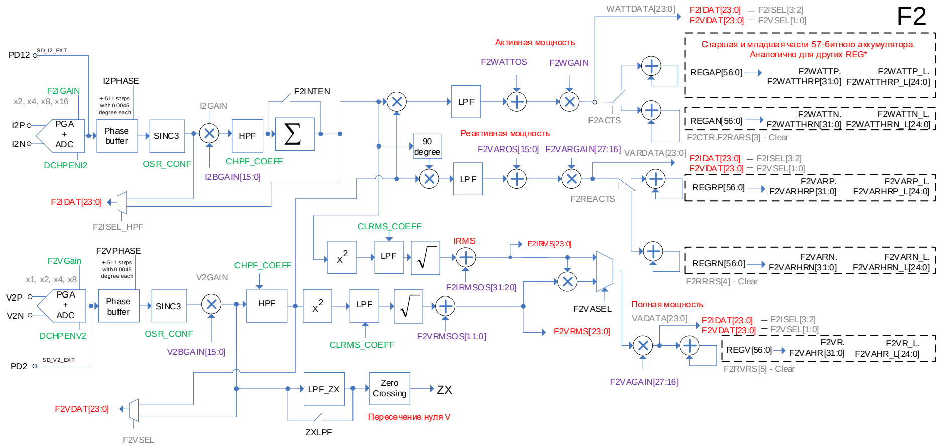
Рисунок 29 – Структурная схема F2
