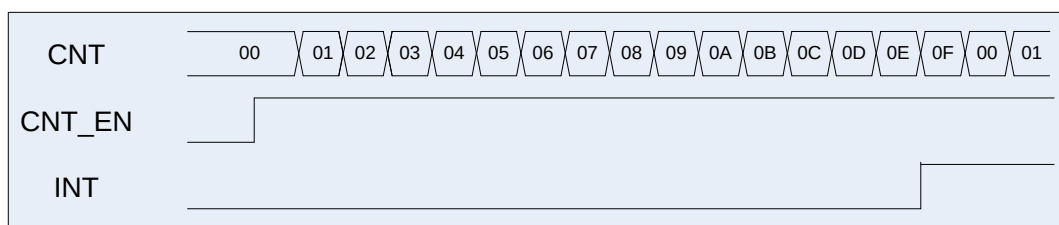
Рисунок 71 – Режим обычного счетчика
