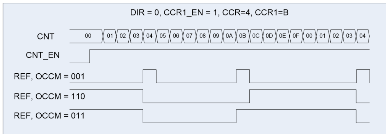
Рисунок 65 – Диаграмма работы в режиме ШИМ, CCR1_EN = 1
