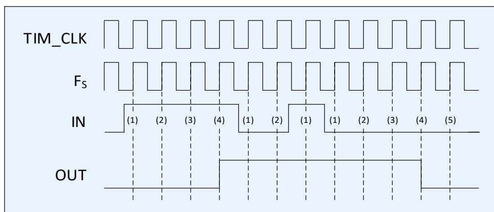
Рисунок 69 – Диаграмма работы фильтра, F_S = \text{TIM\_CLK} , N = 4
