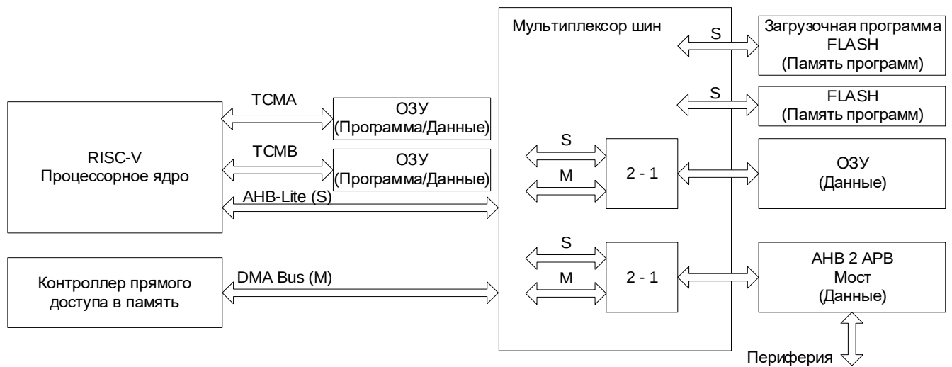
Рисунок 14 – Структурная схема организации памяти
