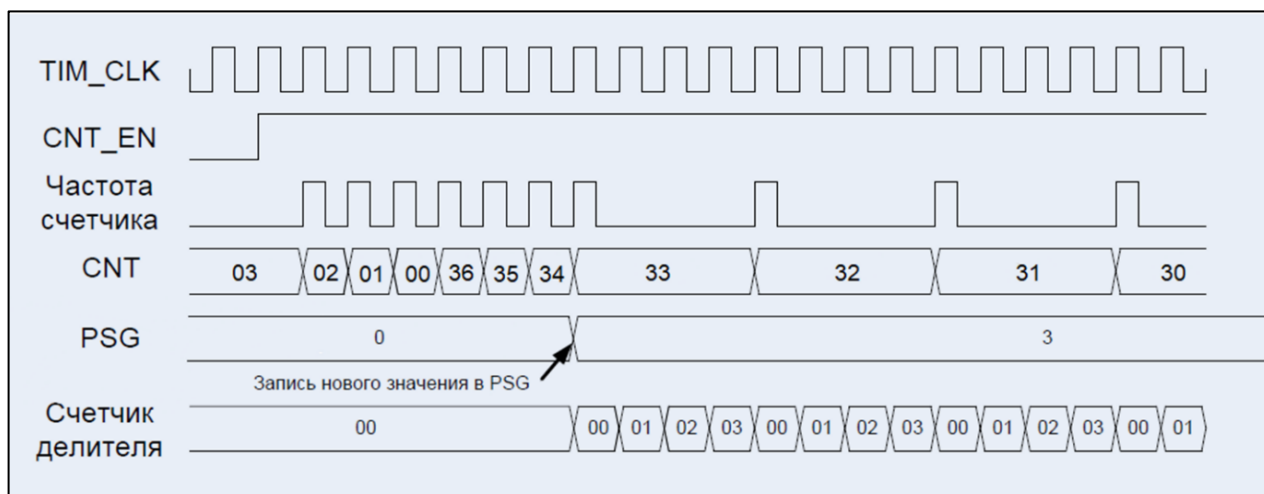
Рисунок 54 – Диаграмма работы счетчика: счет обратный (CNT_MODE[1:0] = 00, EVNT_SEL[3:0] = 0000, DIR = 1)
