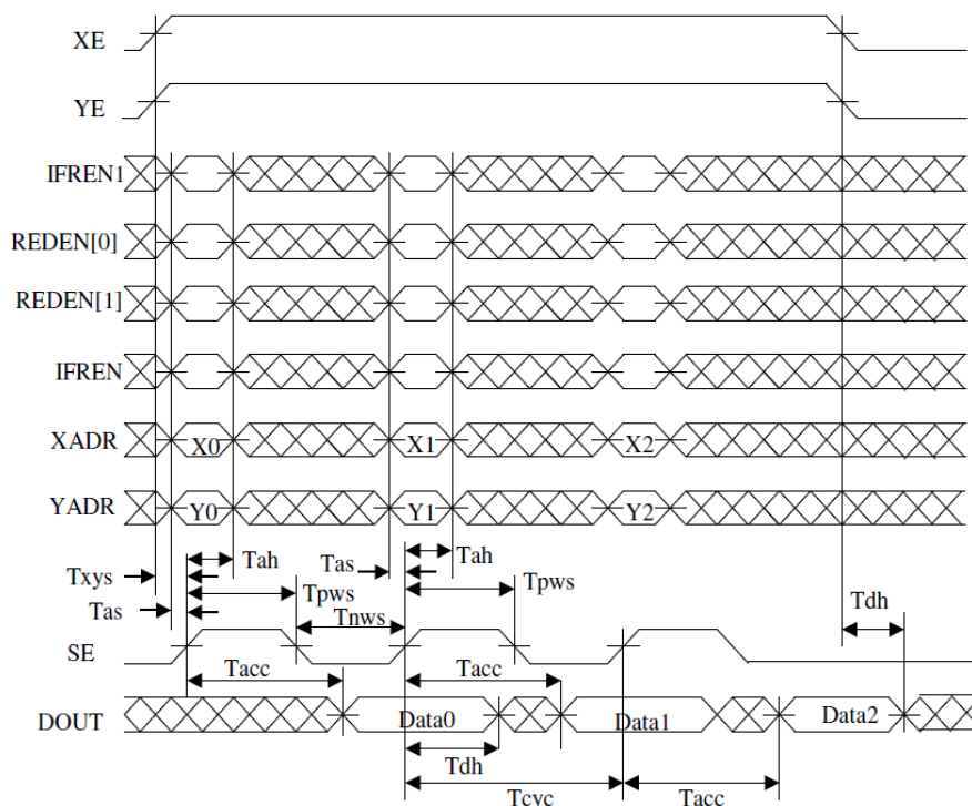
Рисунок 20 – Временная диаграмма чтения памяти
