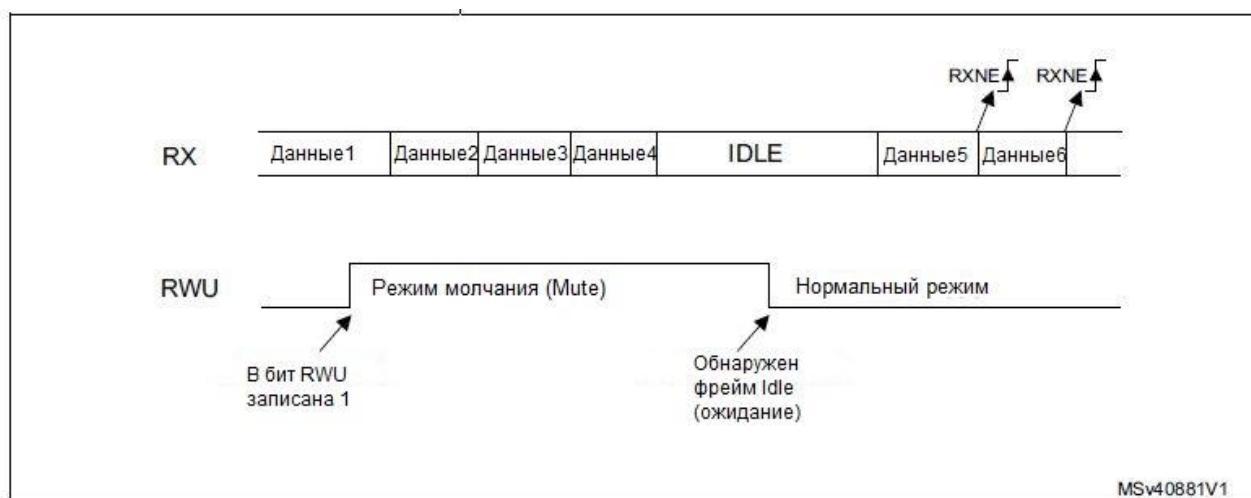
Рисунок 126 – Режим молчания (Mute) с обнаружением линии Idle
