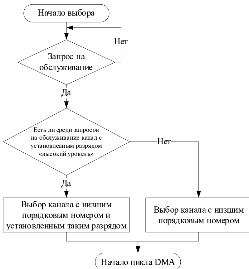
Рисунок 106 – Алгоритм выбора следующего канала для обслуживания
