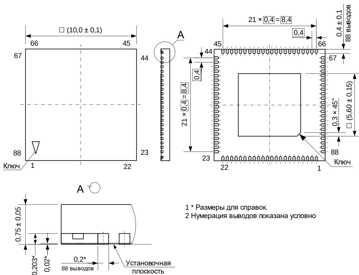
Рисунок 150 – Микросхемы MDR1206FI, MDR1206AFI в корпусе QFN88 10×10×0,75 (0,4)
