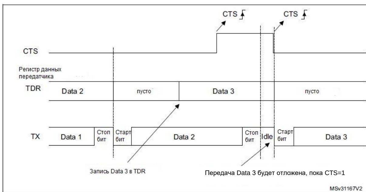
Рисунок 136 – Управление потоком CTS
