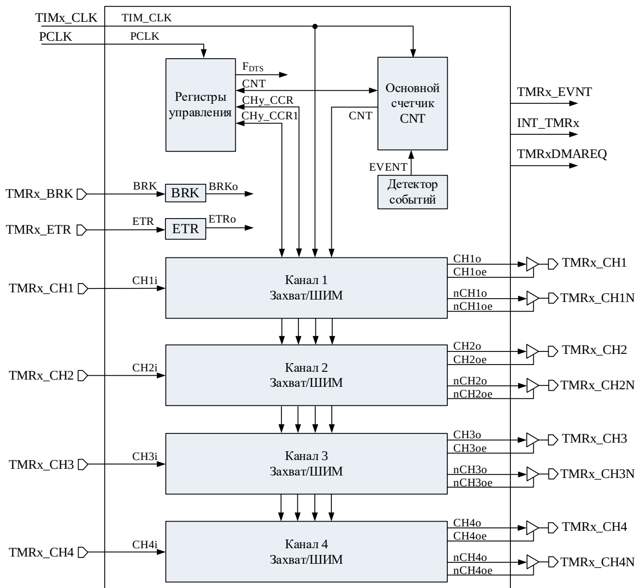
Рисунок 45 – Структурная схема блока «Таймер»
