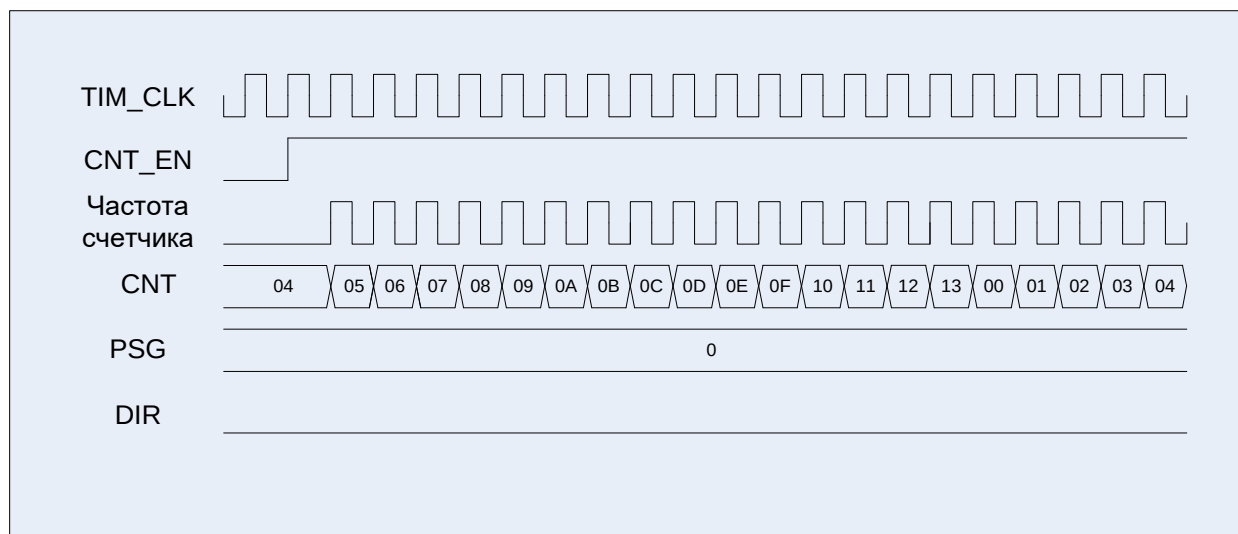
Рисунок 46 – Диаграммы работы таймера, счет прямой от 0 до 0x13, стартовое значение 0x04
