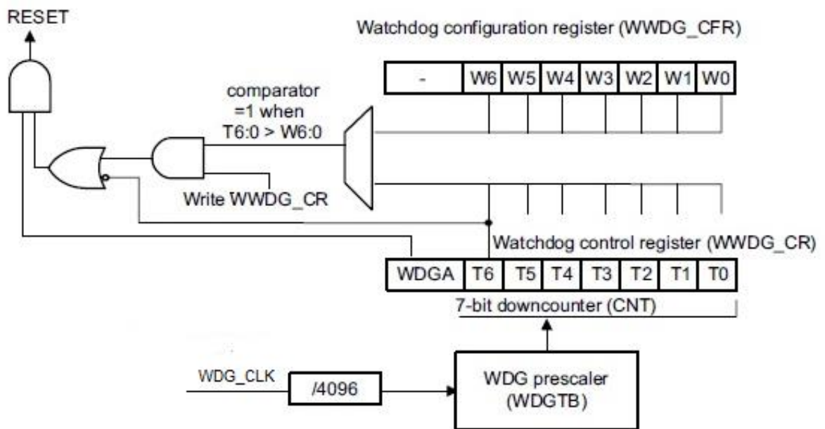
Рисунок 116 – Блок-схема оконного сторожевого таймера
