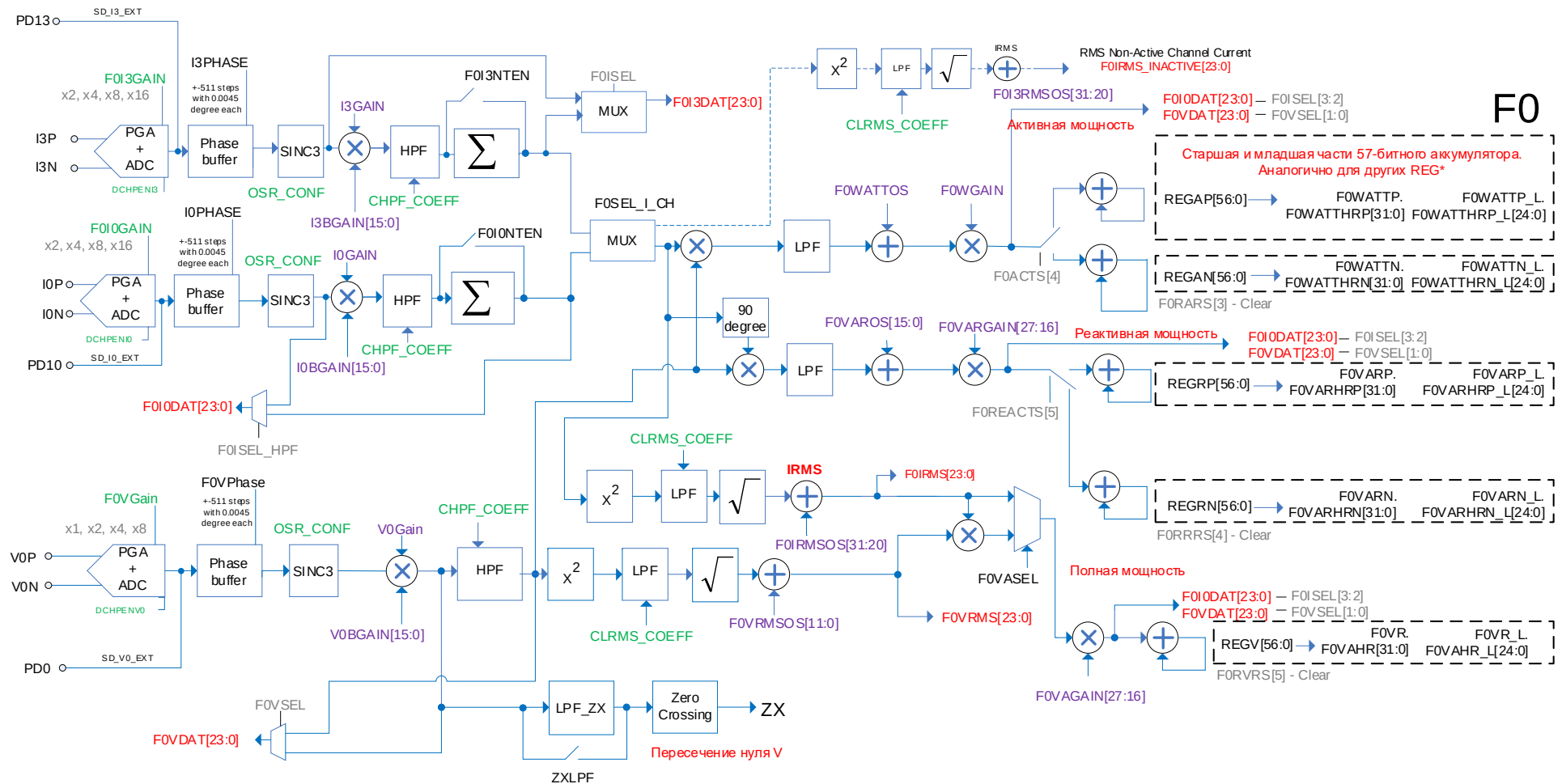
Рисунок 27 – Структурная схема F0
