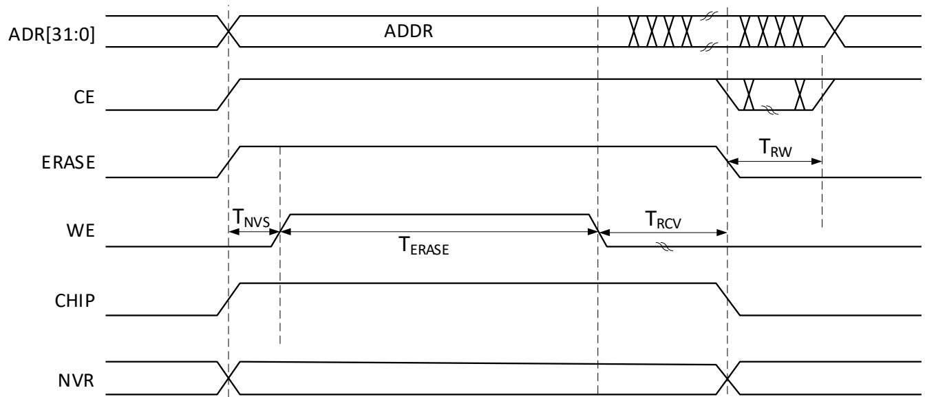
Рисунок 22 – Временная диаграмма стирания памяти
