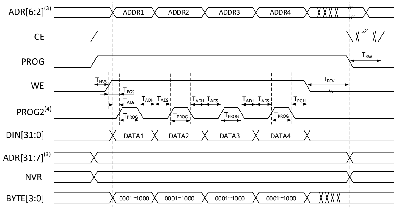
Рисунок 24 – Временная диаграмма записи памяти
