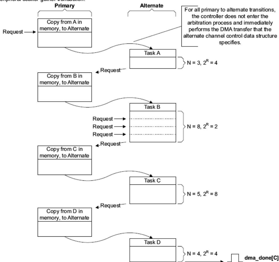
Рисунок 109 – Пример работы DMA в режиме с «Исполнением с изменением конфигурации»
