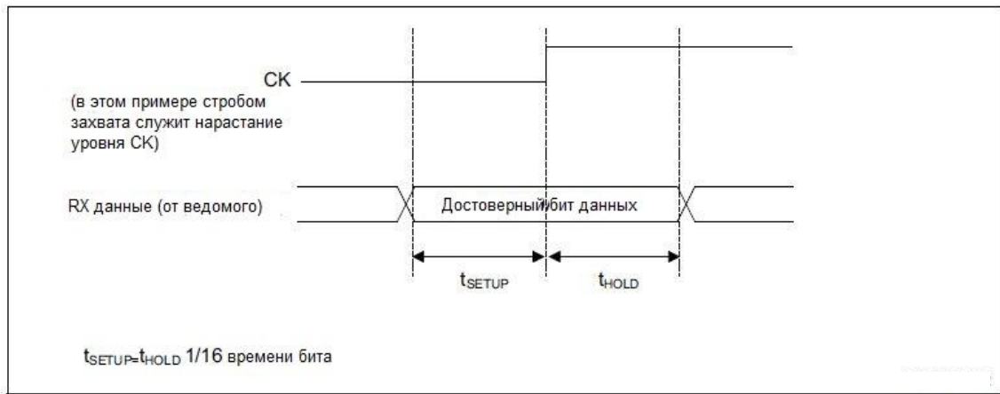
Рисунок 131 – Время установки/удержания RX
