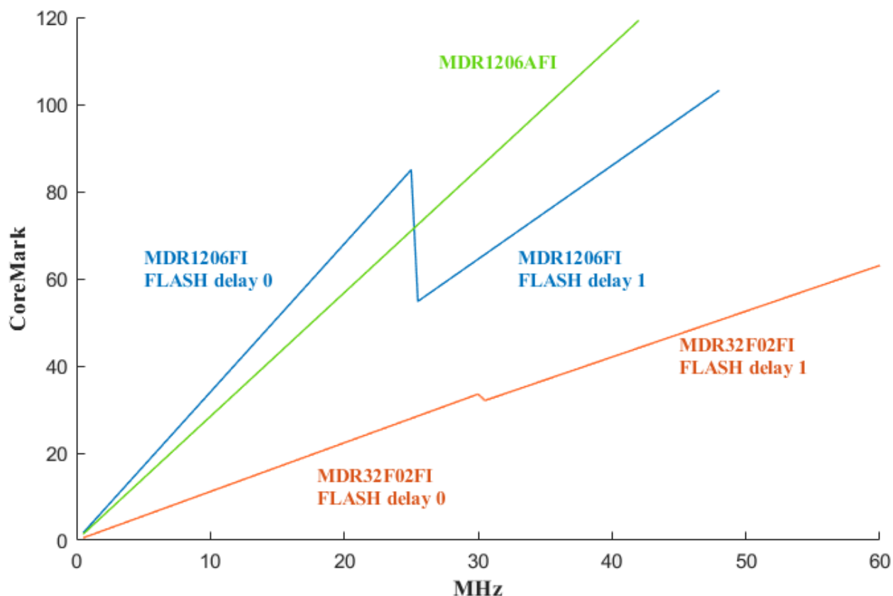
Рисунок 140 – Производительность в Coremark при выполнении из Flash-памяти
