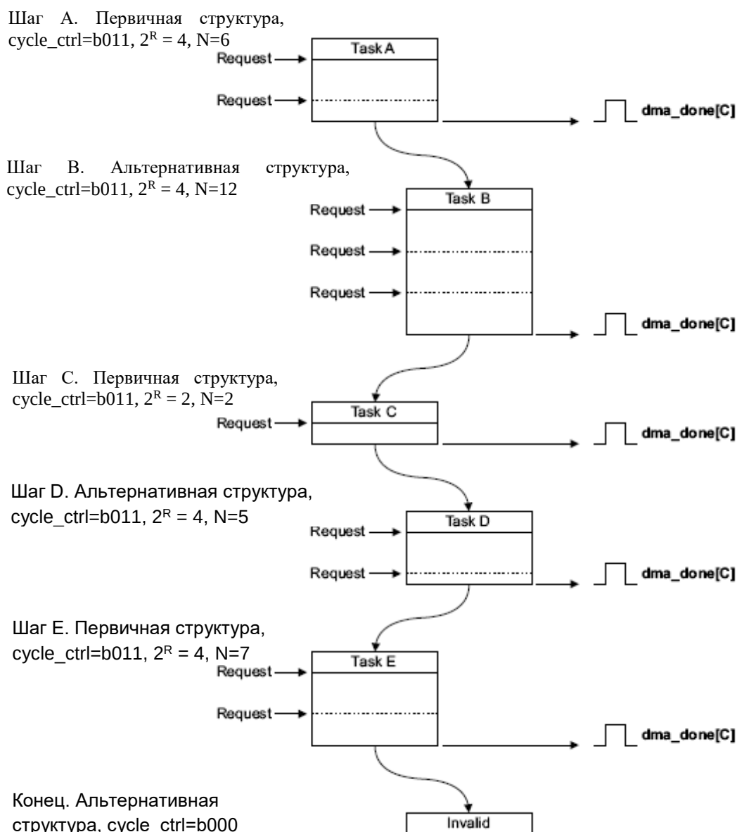
Рисунок 107 – Пример функционирования контроллера в режиме «пинг-понг»
