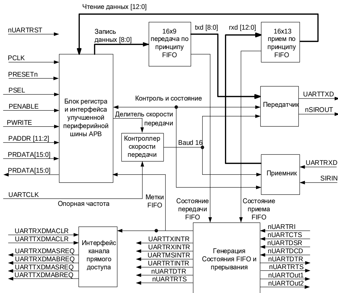
Рисунок 93 – Блок-схема универсального асинхронного приёмопередатчика (UART)
