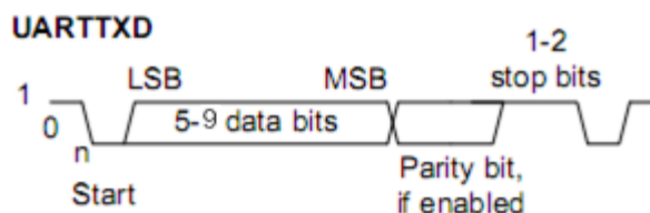
Рисунок 96 – Кадр передачи данных
