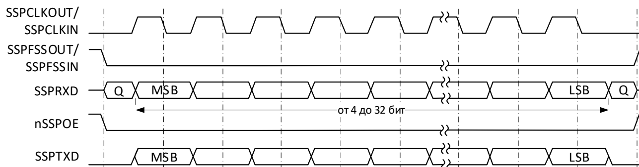
Рисунок 82 – Формат синхронного обмена протокола SPI, SPO=0, SPH=1
