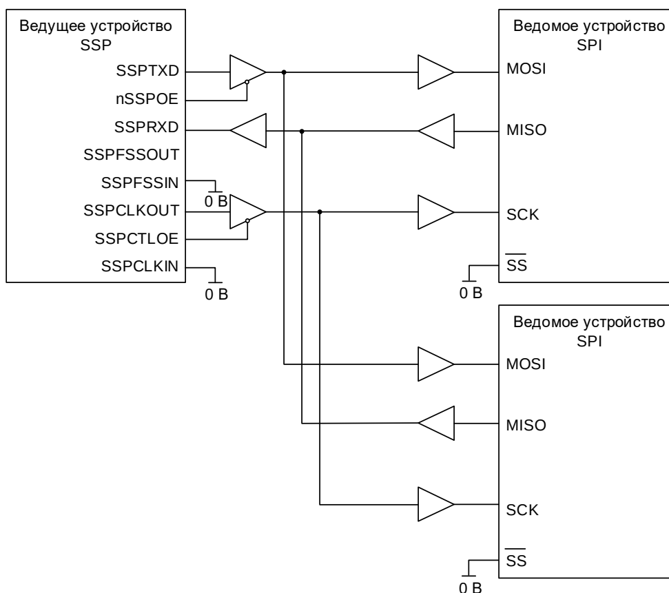
Рисунок 90 – Ведущее устройство SSP подключено к двум ведомым, поддерживающим SPI
