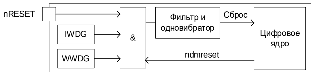
Рисунок 12 – Блок-схема формирования сброса
