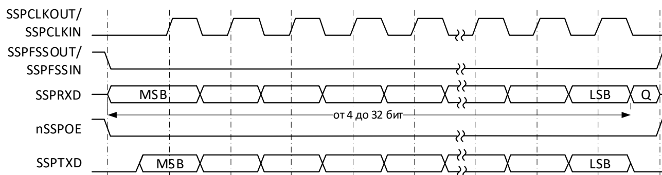
Рисунок 80 – Формат синхронного обмена протокола SPI, SPO=0, SPH=0 (одиночный обмен)
