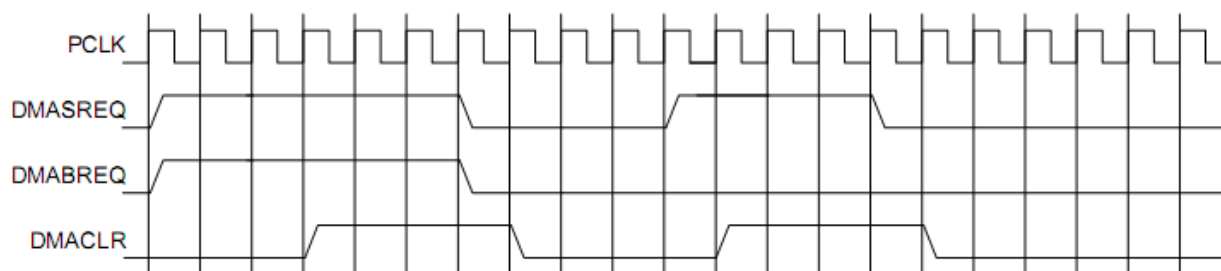
Рисунок 99 – Временные диаграммы одноэлементного и блочного запросов DMA
