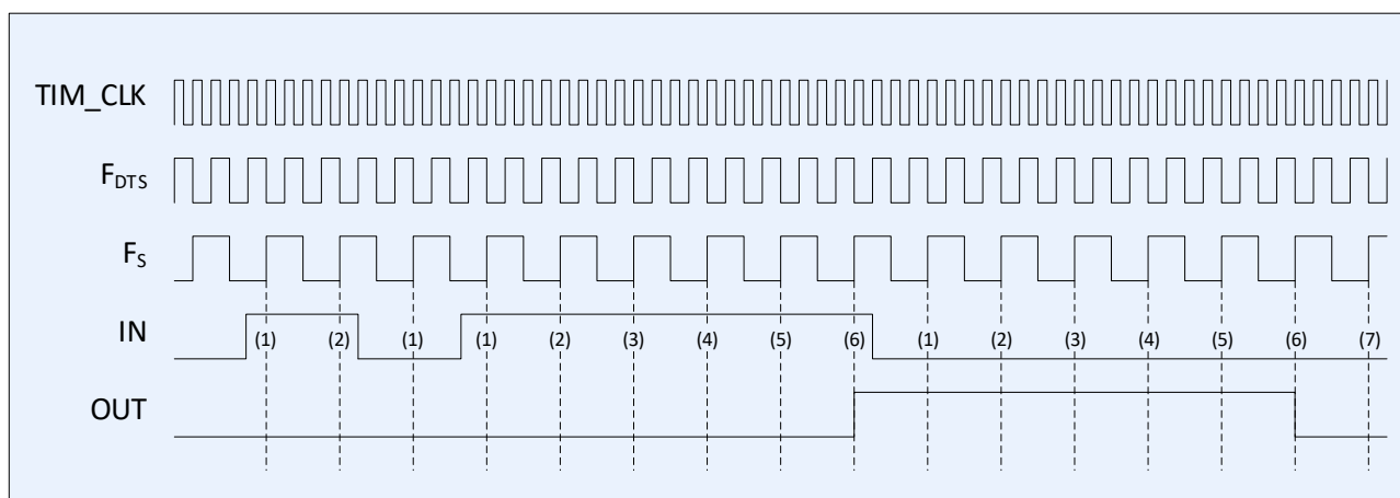
Рисунок 70 – Диаграмма работы фильтра, F_S = F_{DTS}/2 , N = 6
