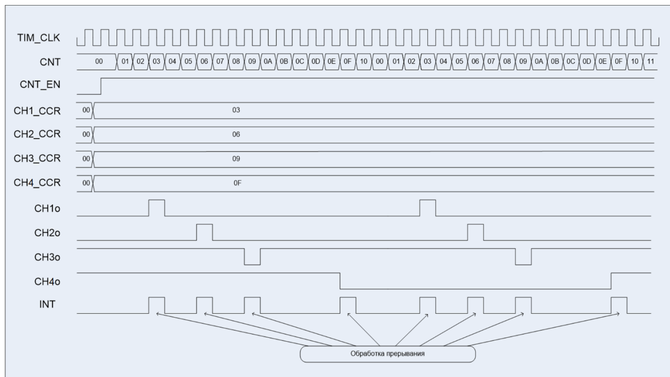
Рисунок 73 – Диаграммы примера работы в режиме ШИМ
