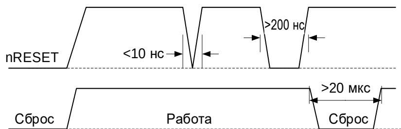
Рисунок 13 – Диаграмма фильтрации помех при формировании сигнала сброса
