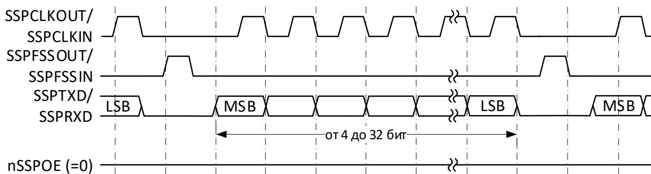
Рисунок 81 – Формат синхронного обмена протокола SPI, SPO=0, SPH=0 (непрерывный обмен)
