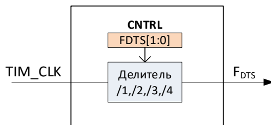
Рисунок 50 – Схема формирования тактовой частоты F DTS
