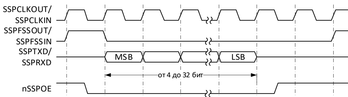
Рисунок 78 – Формат синхронного обмена протокола SSI (единичный обмен)
