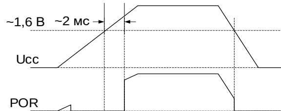
Рисунок 11 – Диаграмма формирования сигнала сброса микросхемы
