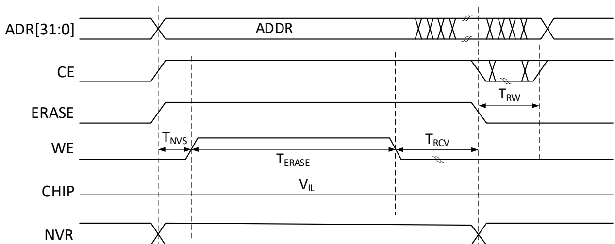
Рисунок 23 – Временная диаграмма стирания страницы памяти
