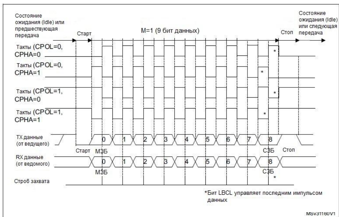
Рисунок 130 – Диаграмма тактирования данных USART (M=1)
