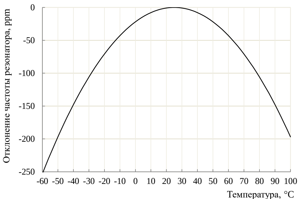
Рисунок 43 – Типовая зависимость отклонения частоты кварцевого резонатора 32 кГц от температуры
