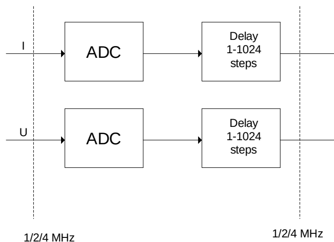
Рисунок 33 – Контролируемый фазовый сдвиг в каналах тока и напряжения
