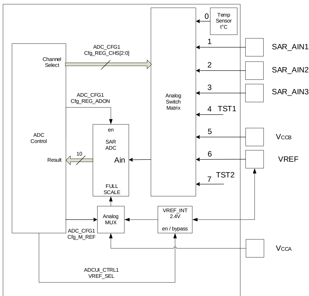
Рисунок 74 – Структурная схема АЦП
