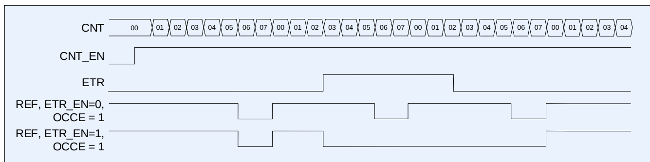
Рисунок 66 – Диаграмма сброса сигнала REF по выводу ETR
