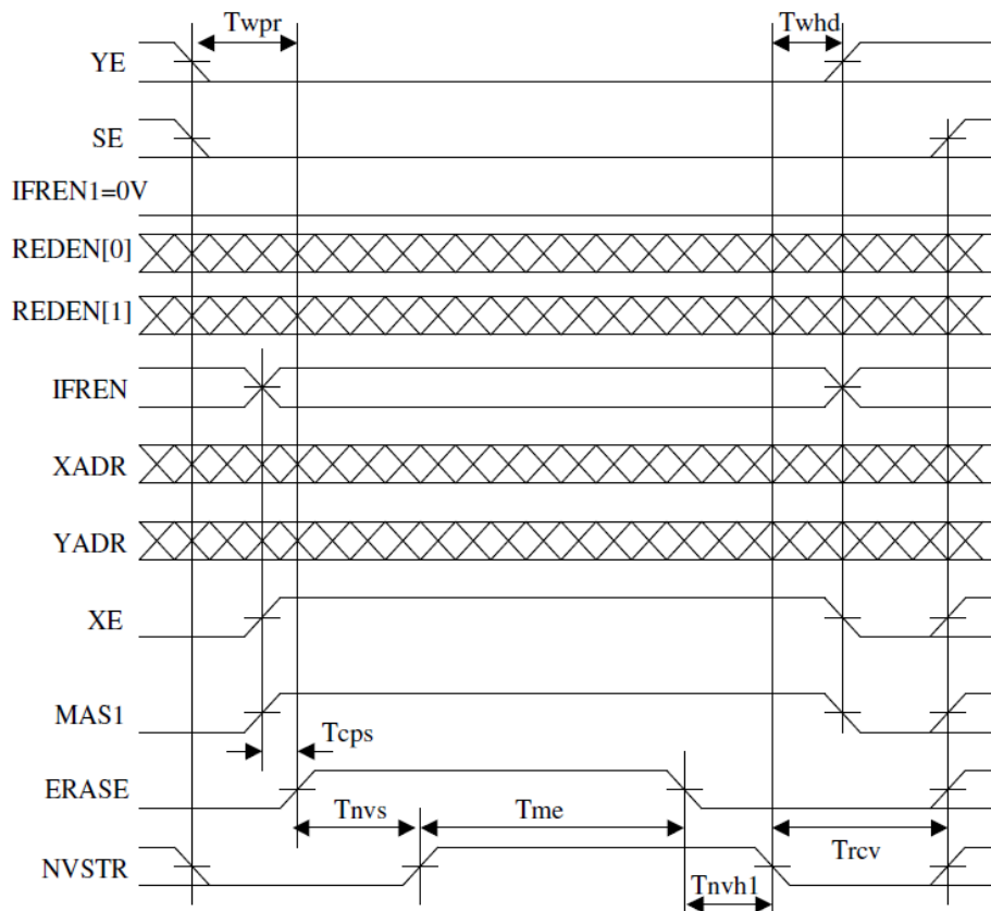
Рисунок 17 – Временная диаграмма стирания памяти
