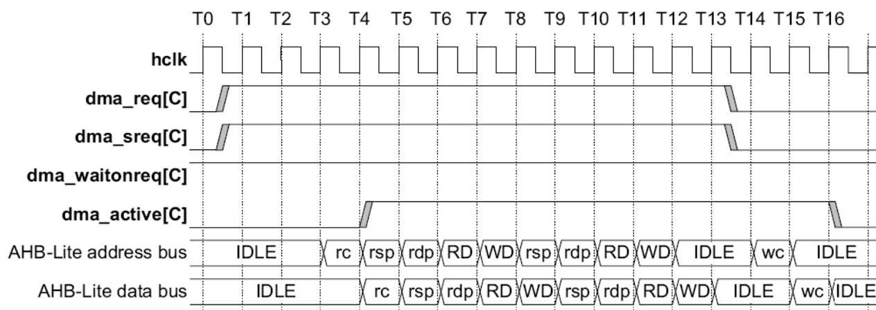
Рисунок 104 – Диаграмма работы контроллера DMA при использовании dma_waitonreq
