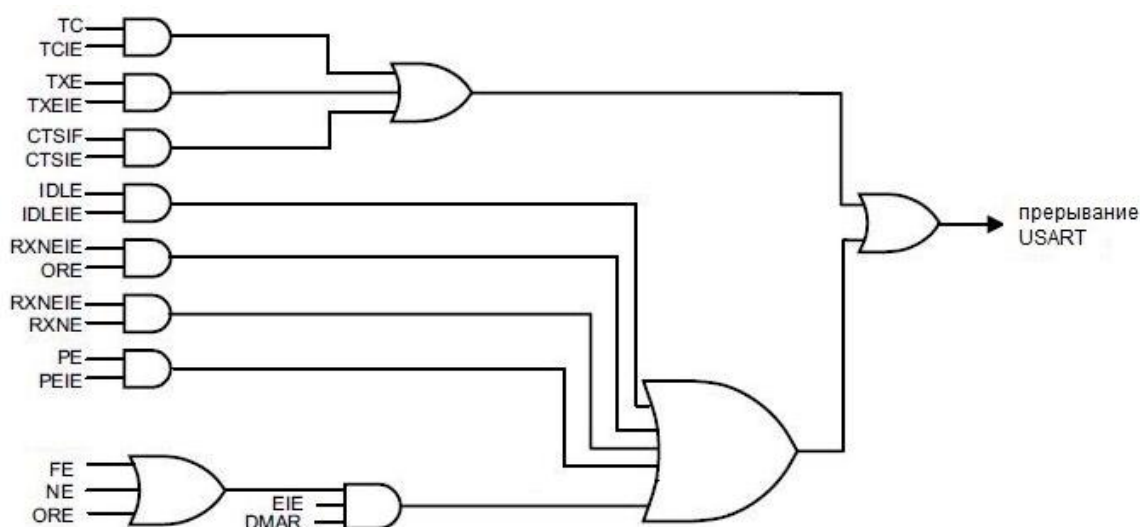
Рисунок 137 – Диаграмма отображений событий USART на прерывание
