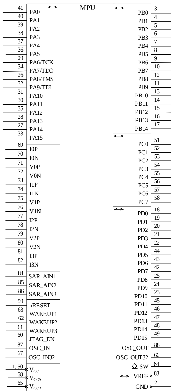
Рисунок 3 – Условное графическое изображение микросхем MDR1206FI, MDR1206AFI
