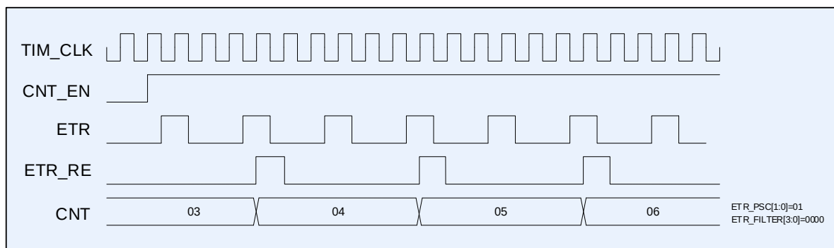
Рисунок 60 – Диаграмма тактирования со входа ETR, EVNT\_SEL[3:0] = 1000
