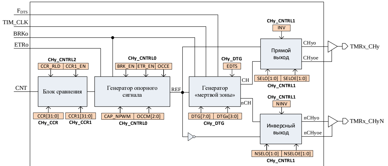
Рисунок 63 – Структурная схема блока формирования ШИМ
