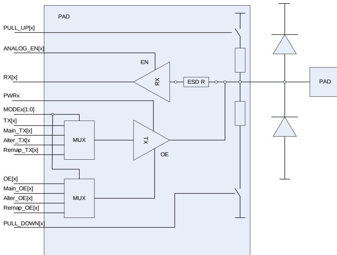
Рисунок 44 – Блок схема разряда порта ввода-вывода
