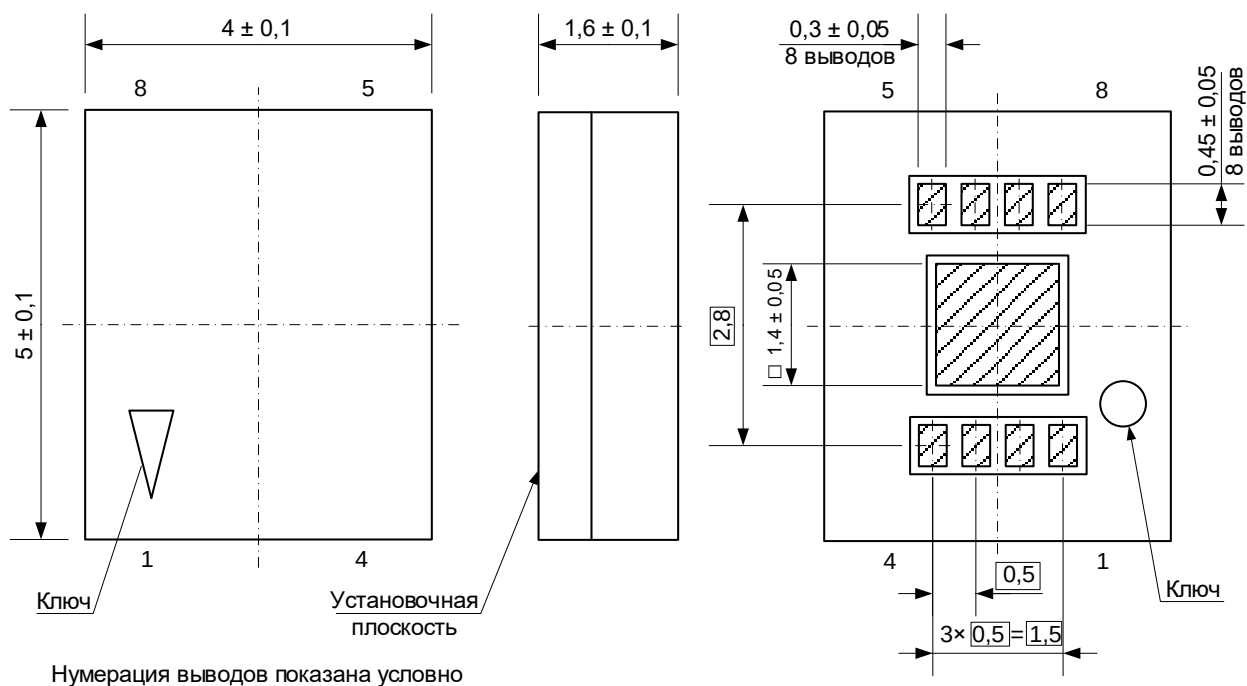
Рисунок 151 – Микросхемы MDR1215LGI в корпусе LGA8 4×5×1,6 (0,5)
