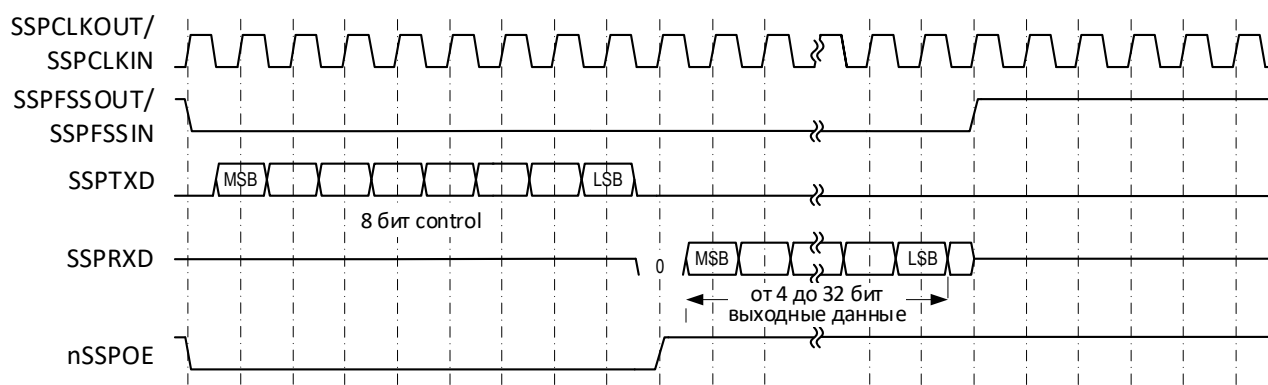
Рисунок 86 – Формат синхронного обмена протокола Microwire (одиночный обмен)
