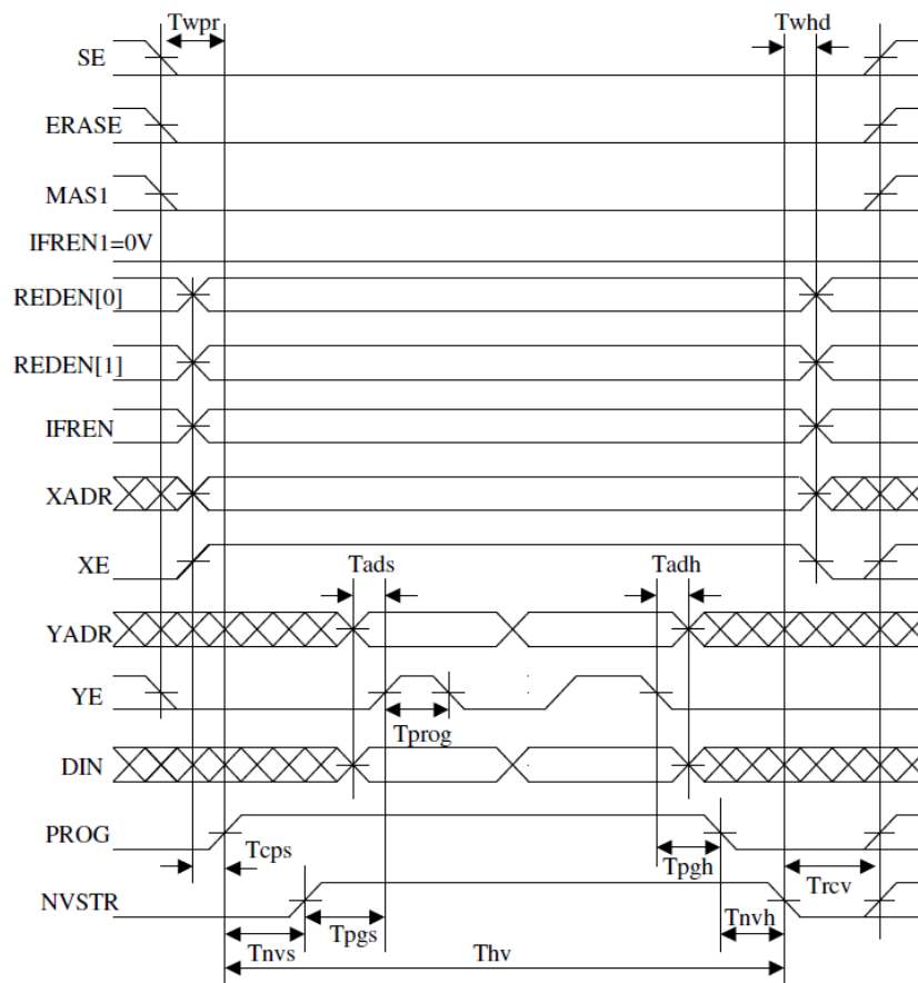
Рисунок 19 – Временная диаграмма записи памяти
