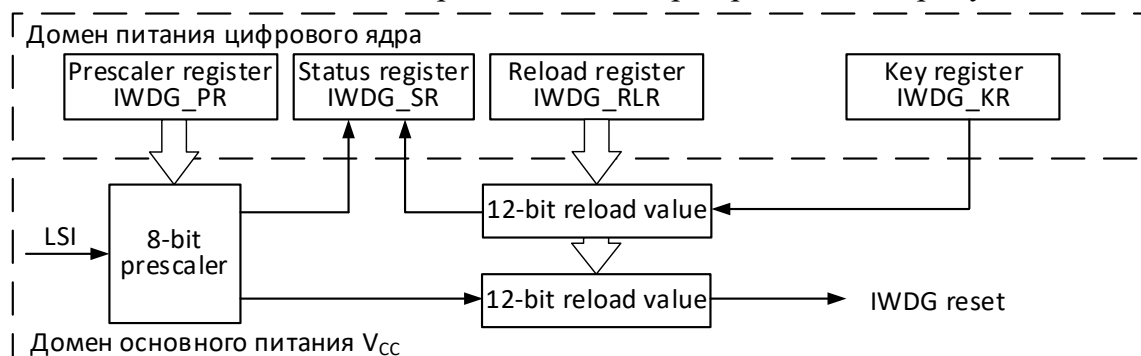
Рисунок 115 – Блок-схема независимого сторожевого таймера
