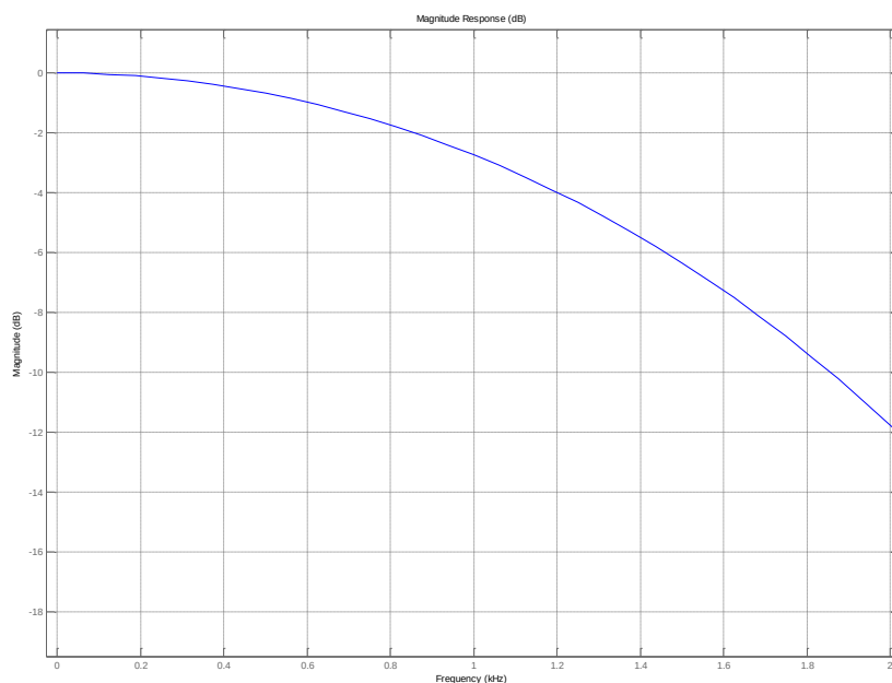
Рисунок 34 – Характеристика децимирующего фильтра в полосе 2 кГц
