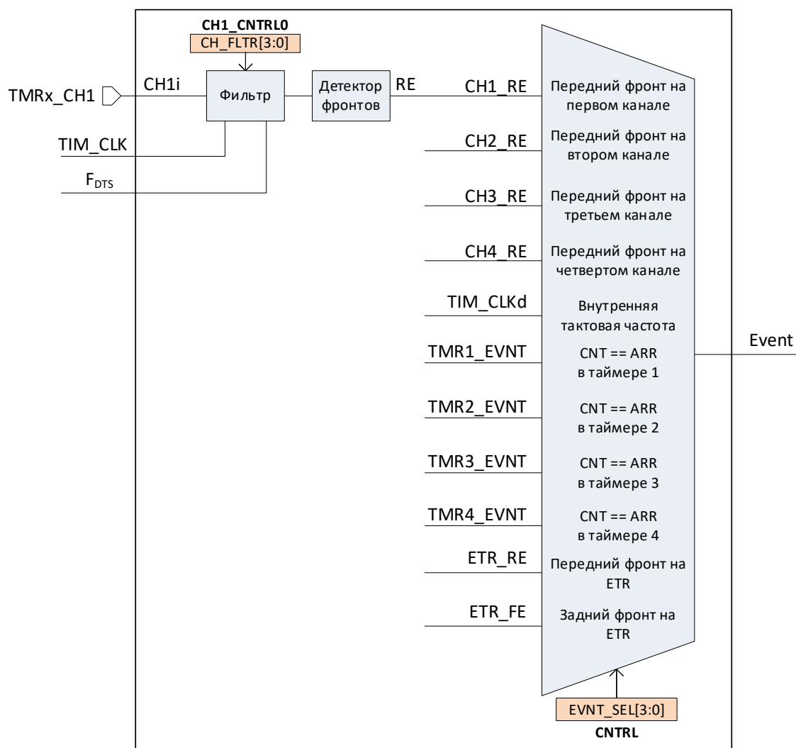
Рисунок 57 – Схема тактирования сигналом со входа первого канала
