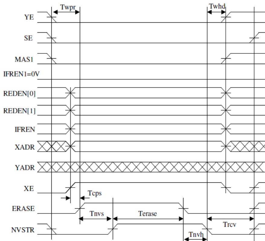
Рисунок 18 – Временная диаграмма стирания страницы памяти
