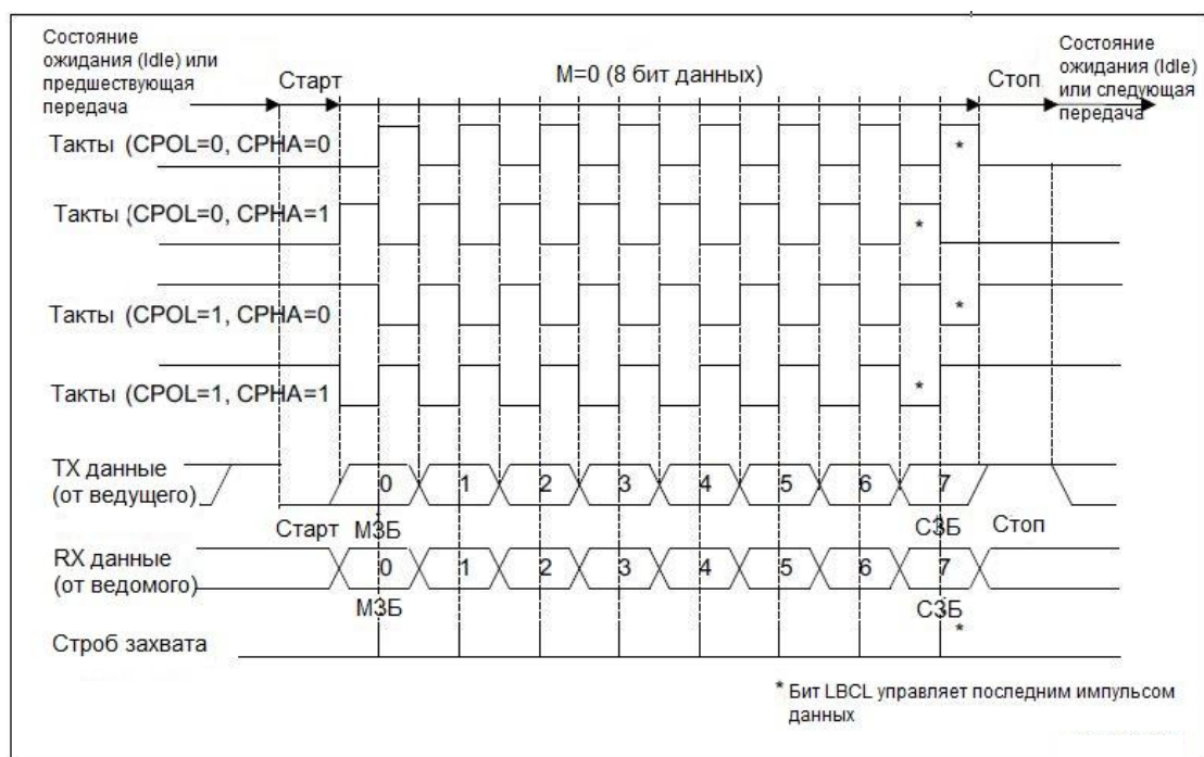
Рисунок 129 – Диаграмма тактирования данных USART (M=0)
