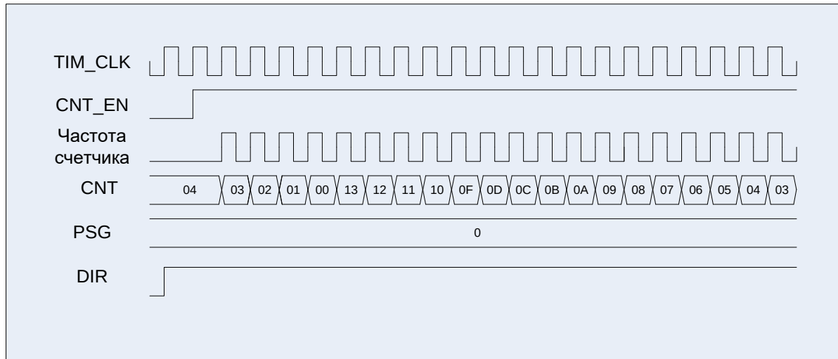
Рисунок 47 – Диаграммы работы таймера, счет обратный от 0x13 до 0, стартовое значение 0x04
