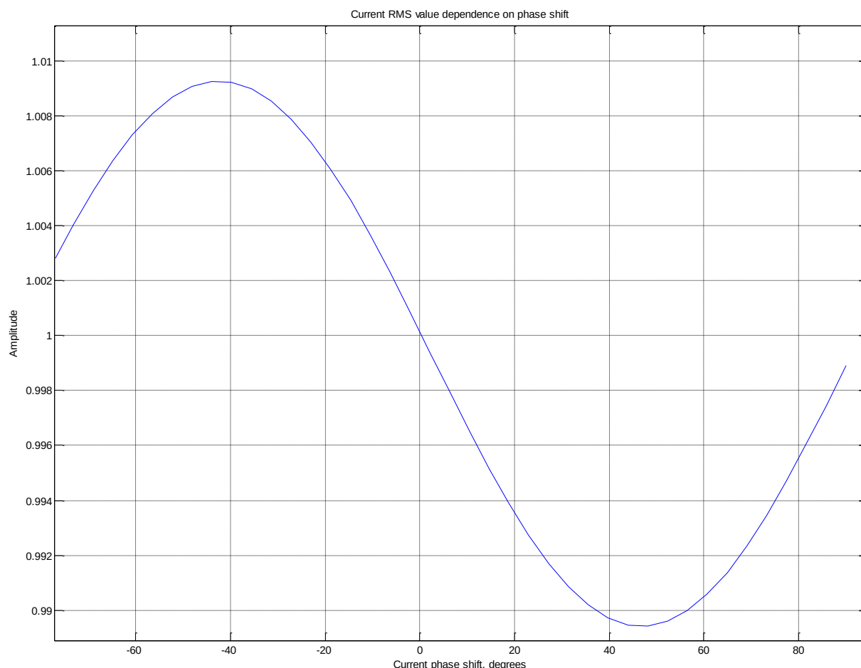
Рисунок 30 – Зависимость RMS от сдвига фазы входного сигнала
