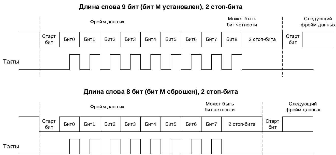
Рисунок 120 – Программирование длины слова
