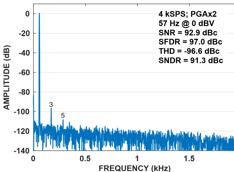
Рисунок 139 – Типовой спектр в НУ для \Delta\Sigma АЦП микросхем MDR1206AFI (CHIP_ID = 215) в канале F2IDAT для дифференциального входного сигнала +/- 1 В (0.707 RMS). Усиление = 6 дБ (F2IGAIN = 00)
