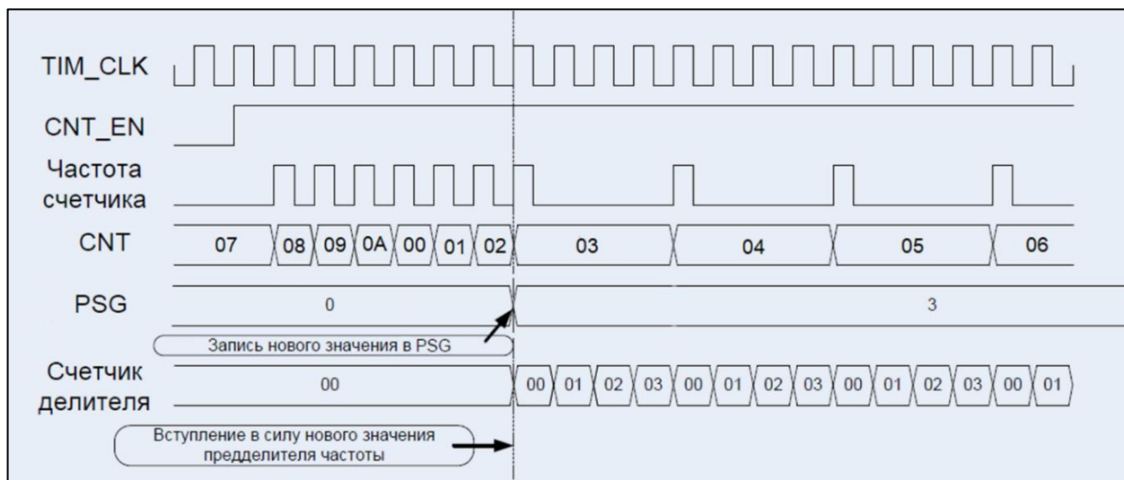
Рисунок 53 – Диаграмма работы счетчика: счет прямой (CNT_MODE[1:0] = 00, EVNT_SEL[3:0] = 0000, DIR = 0)
