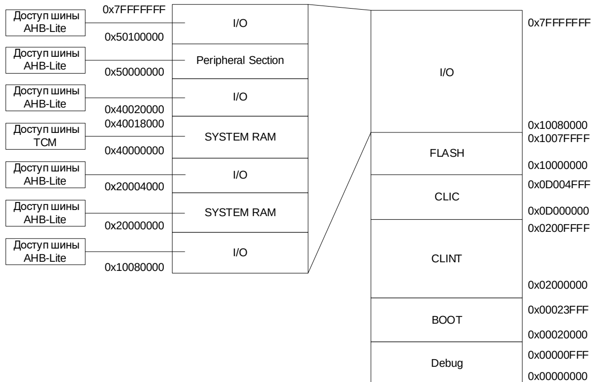
Рисунок 15 – Структура адресного пространства микросхемы
