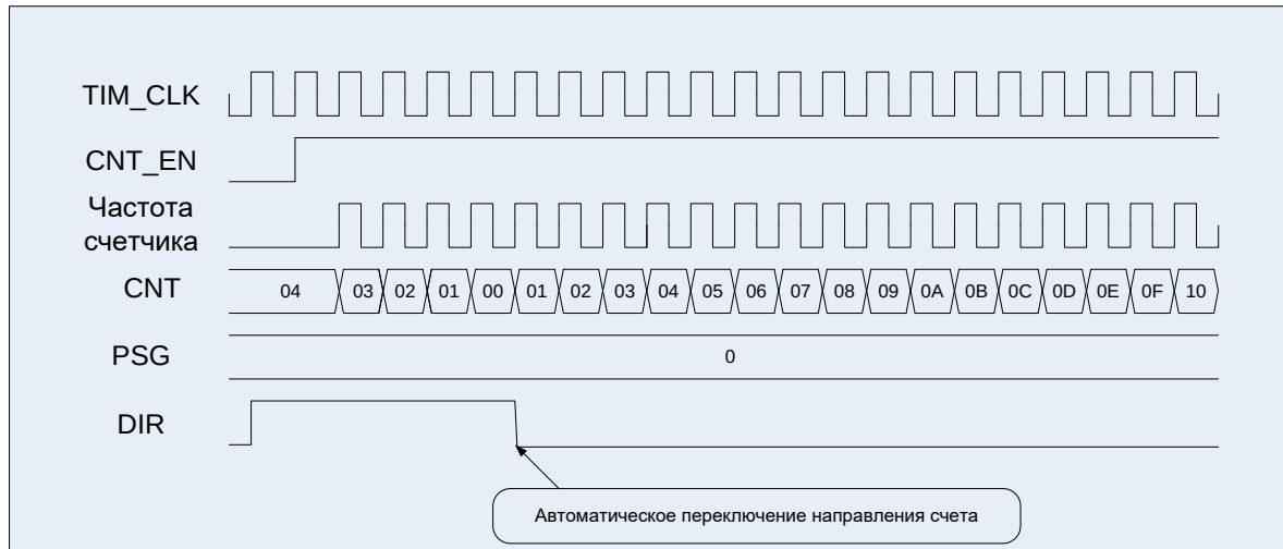
Рисунок 49 – Диаграммы работы таймера, счет двунаправленный, сначала обратный
