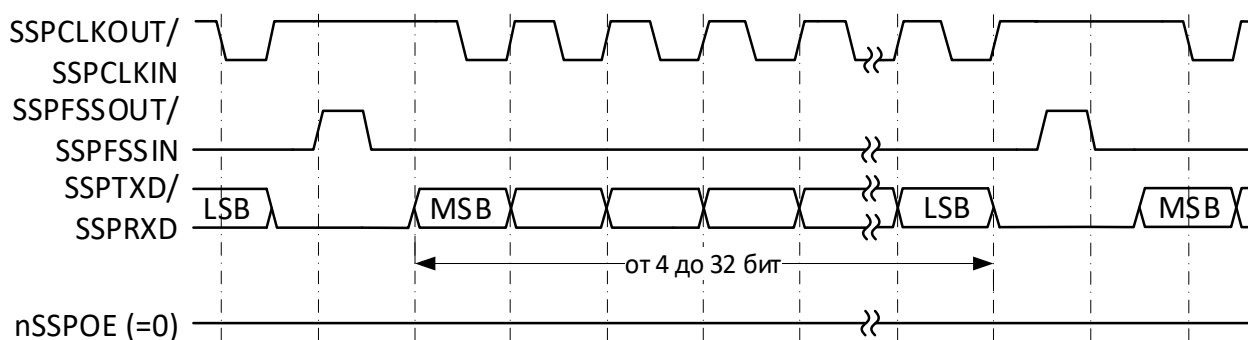
Рисунок 84 – Формат синхронного обмена протокола SPI, SPO=1, SPH=0 (непрерывный обмен)
