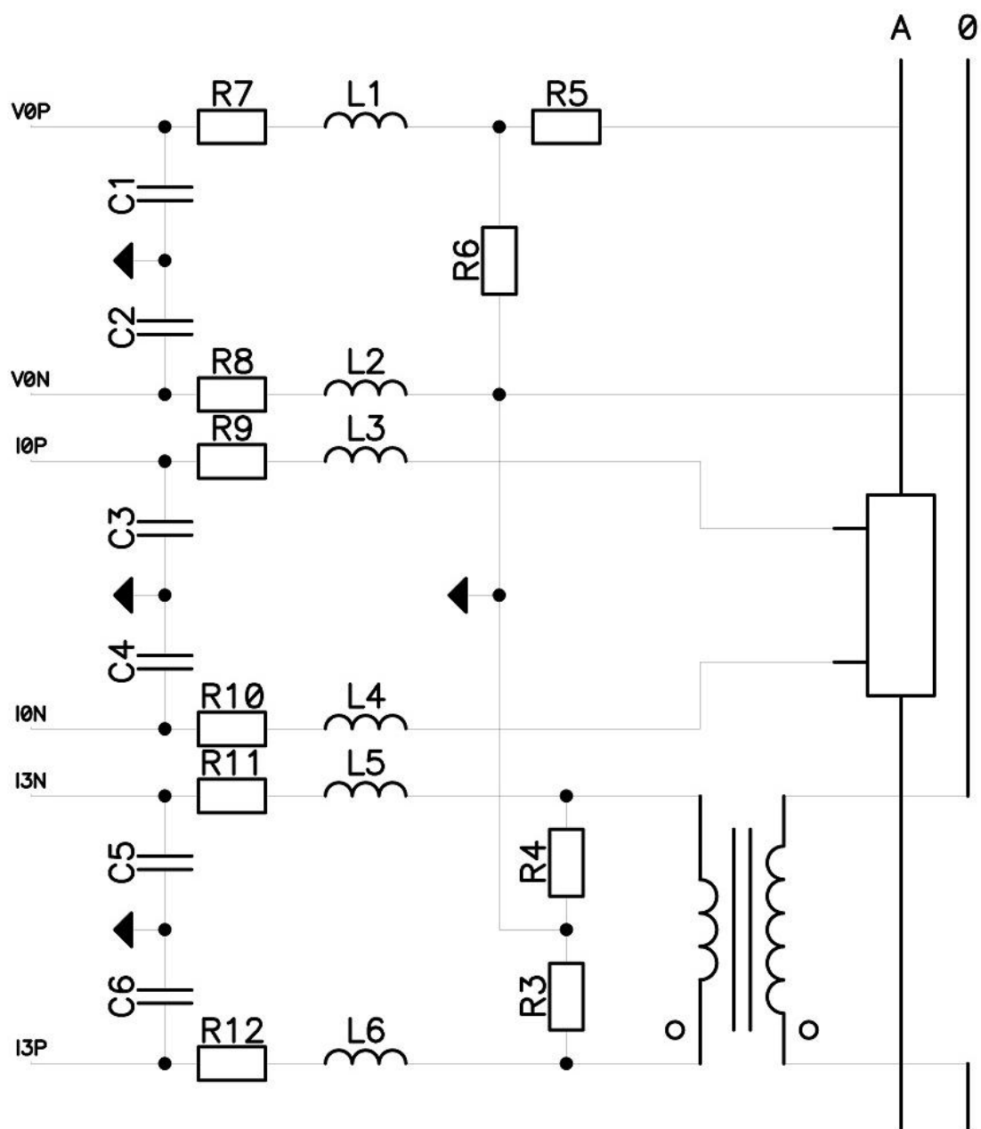
Рисунок 39 – Типовая схема включения для учета электроэнергии по одной фазе с использованием шунта
