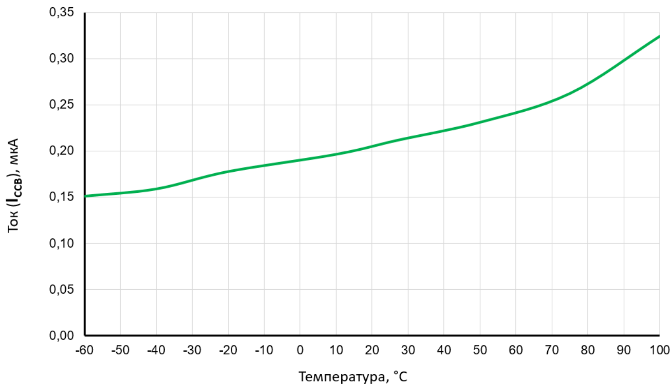
Рисунок 146 – Зависимость статического тока потребления I_{CCB} батарейного домена микросхем MDR1206FI (CHIP_ID = 217) от температуры при U_{CCB} = 3,3 В
