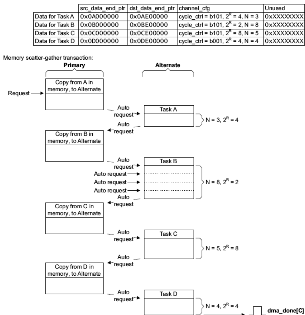
Рисунок 108 – Пример работы DMA в режиме с «Исполнением с изменением конфигурации»
