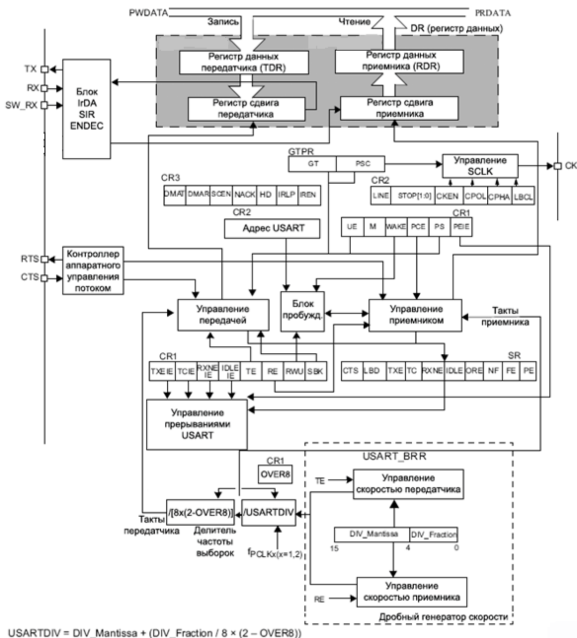
Рисунок 119 – Блок схема USART
