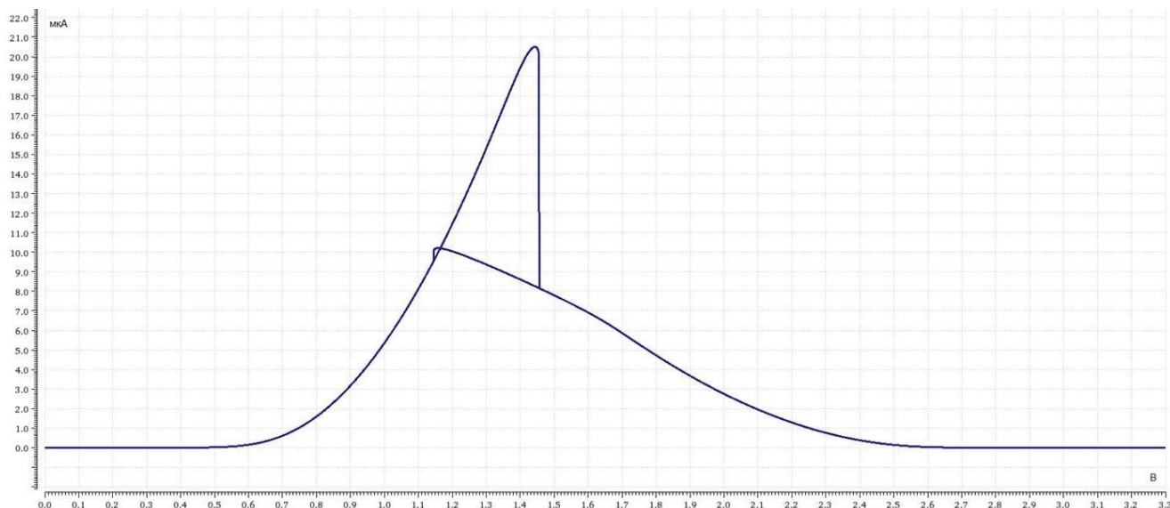
Рисунок 142 – Типовая зависимость дополнительного тока потребления по питанию U_{CCB} от напряжения на входе WAKEUP1-WAKEUP3 при U_{CCB} = 3.3 В в НУ
