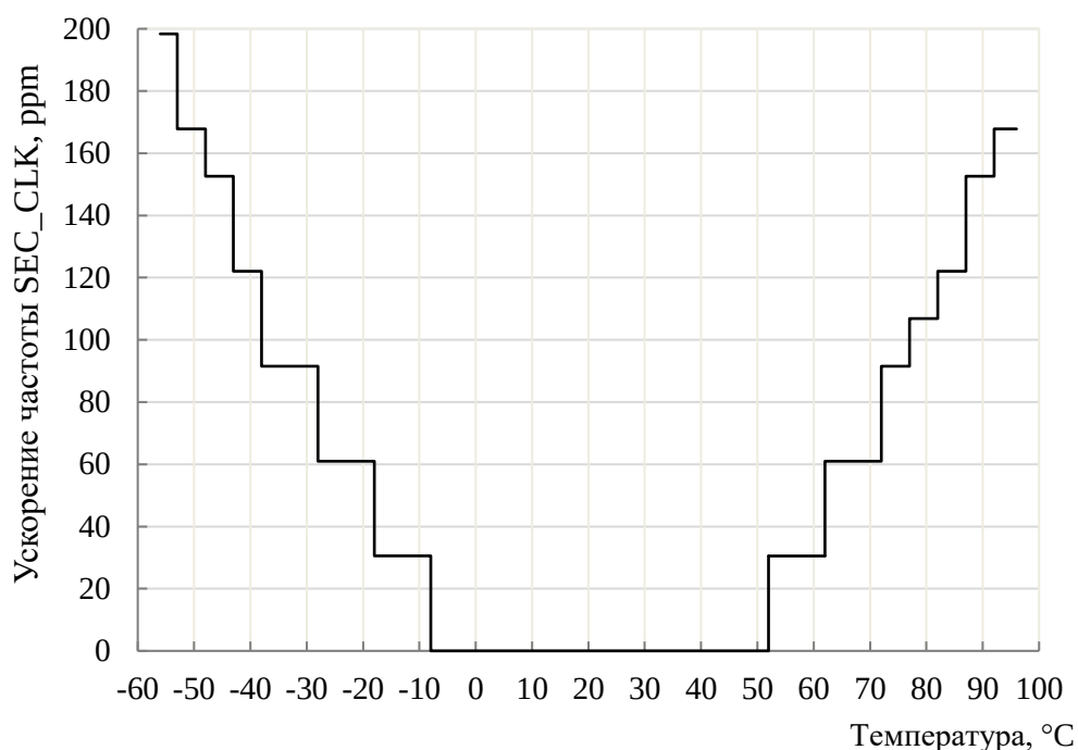
Рисунок 42 – Типовая зависимость поправки (ускорения) частоты SEC_CLK при BKP_RTC_PRL = 32767 от температуры
