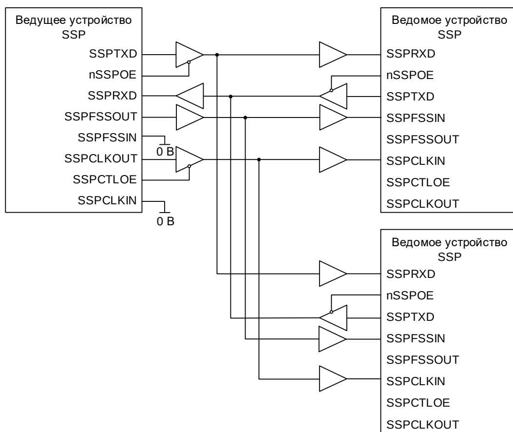
Рисунок 89 – Ведущее устройство SSP подключено к двум ведомым
