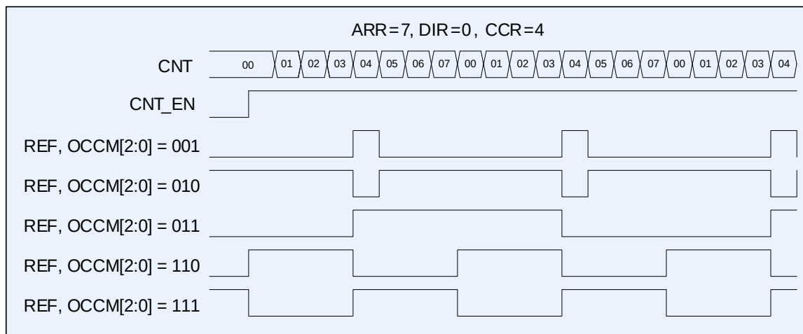
Рисунок 64 – Диаграмма работы в режиме ШИМ, CCR1_EN=0
