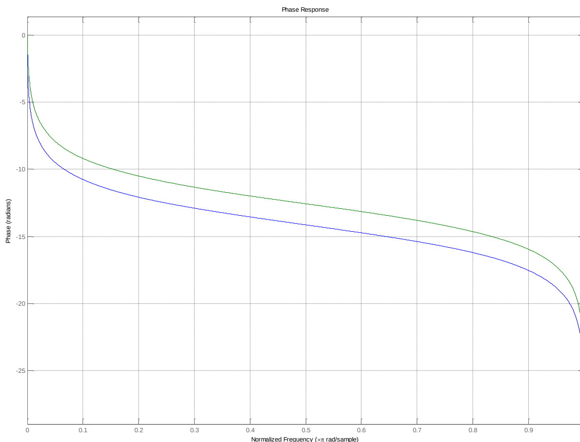
Рисунок 36 – Фильтр для сдвига сигнала на 90 °
