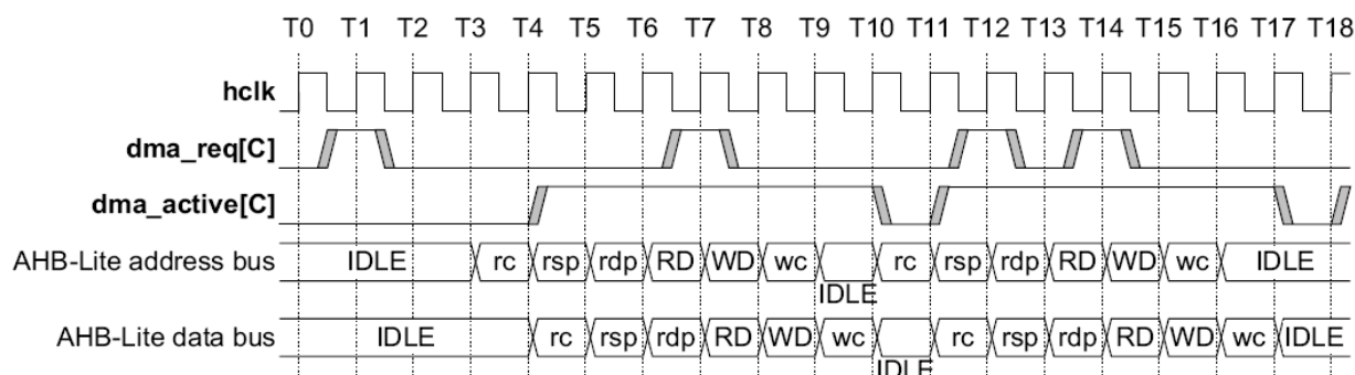
Рисунок 101 – Диаграмма работы при получении импульсного запроса от периферийного блока
