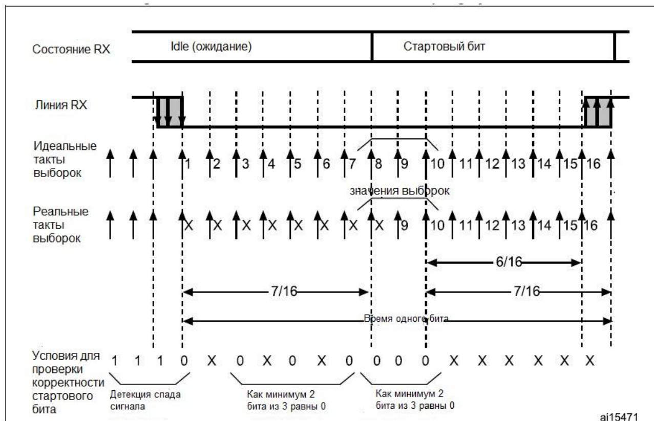
Рисунок 123 – Обнаружение стартового бита при передискретизации на 16 и 8
